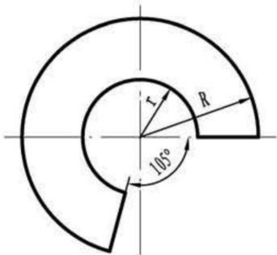
锥形罩展开图
