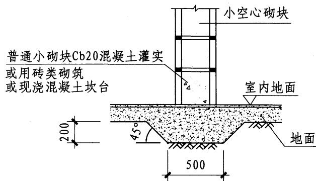
小砌块填充墙体根部做法(三)
