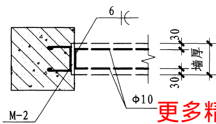
框架柱预埋件
