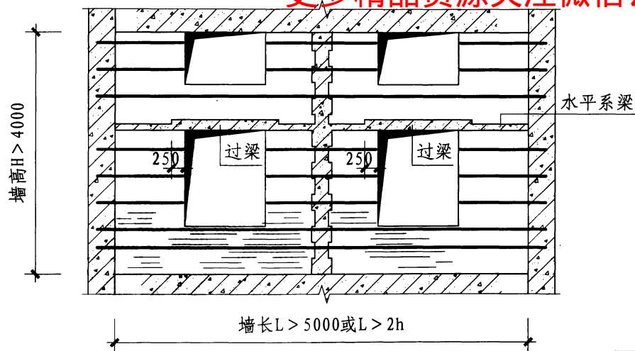
填充墙拉结示意图 (三)
