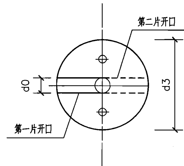
抗力片制作图
