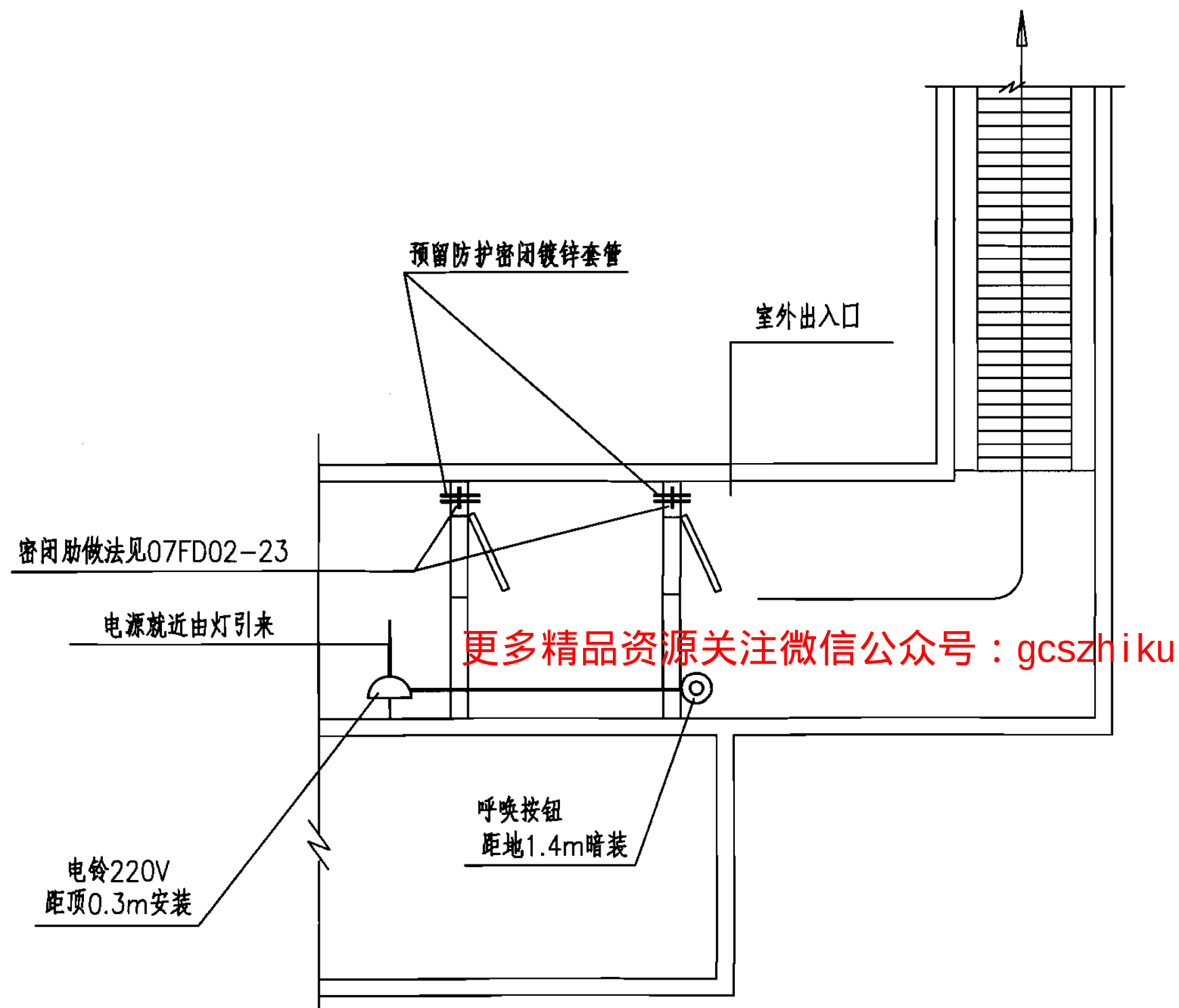
防空地下室出入口普通门铃及按钮布置示例图
