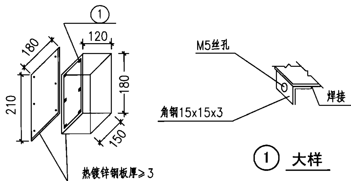
防护密闭接线盒详图
