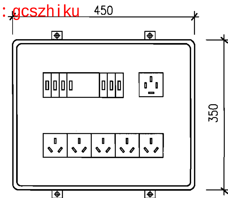
插座箱方案二布置图
