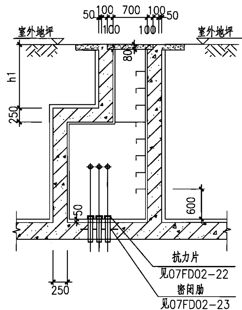
2-2断面
