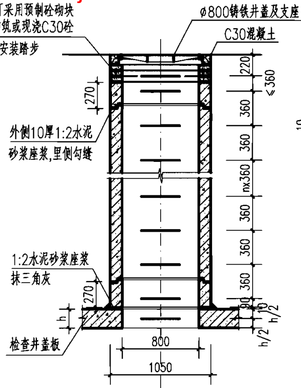
预制井筒安装大样
