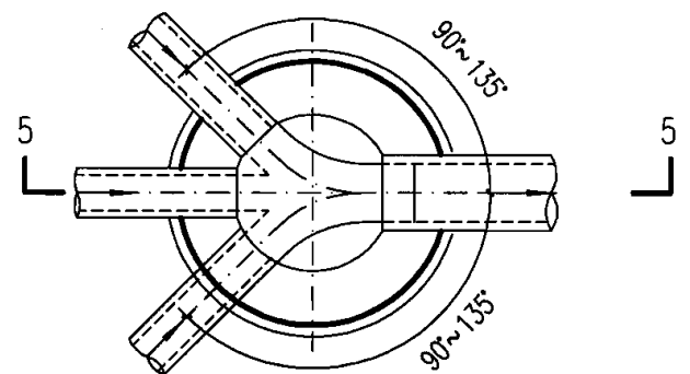
90° ~ 135°四通井平面图
