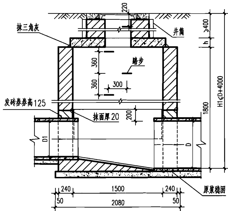
1-1 剖面
