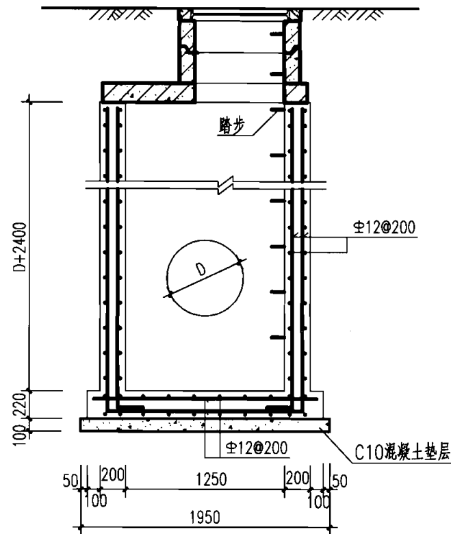
2-2 剖面
