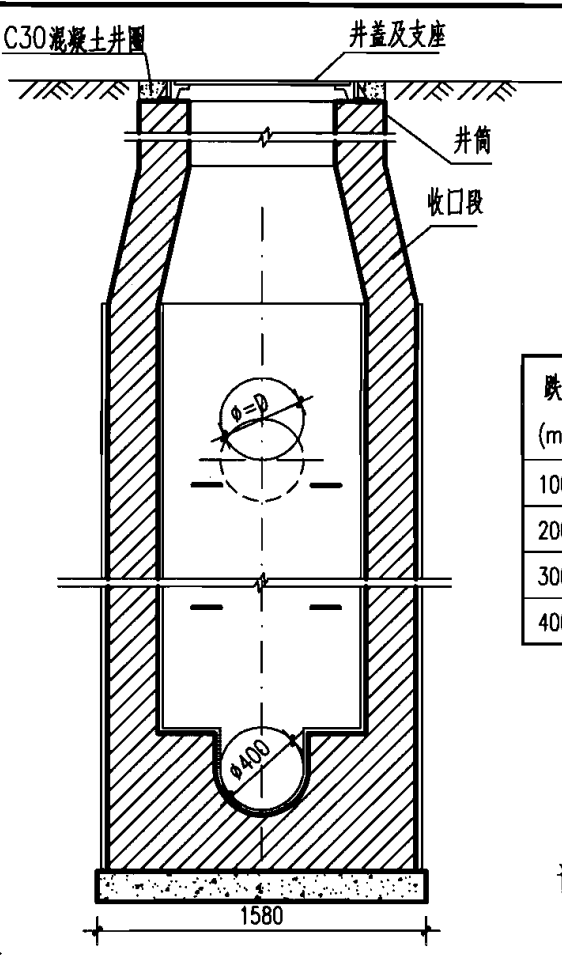
2-2 剖面
