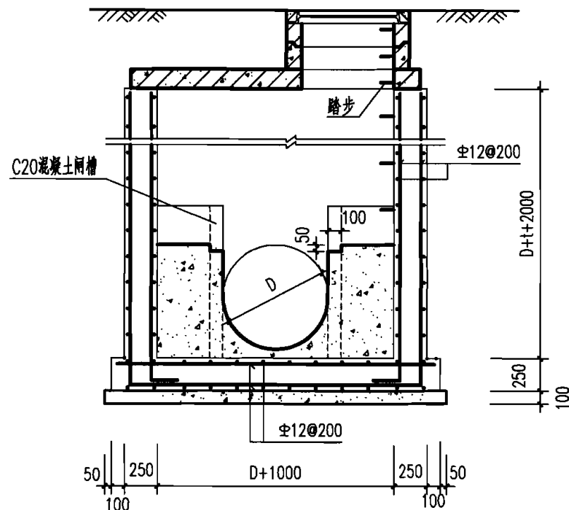
2-2 剖面
