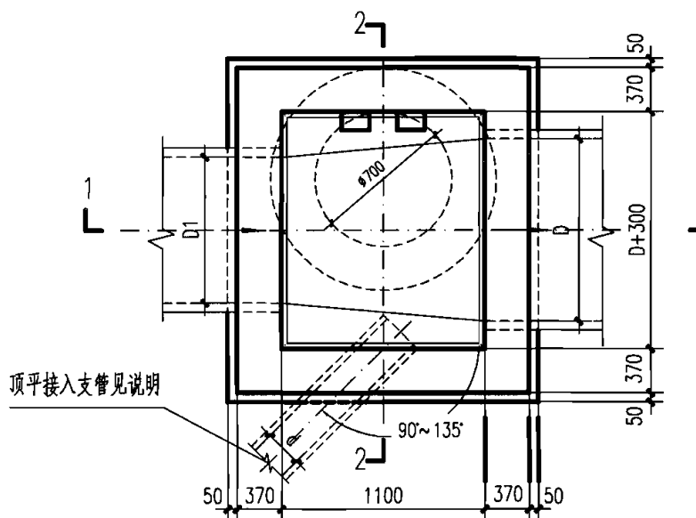
平面图
