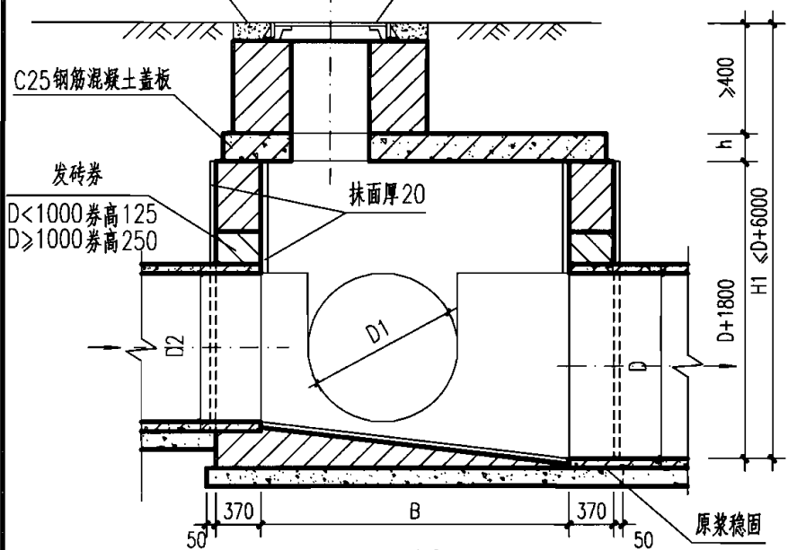
1-1 剖面
