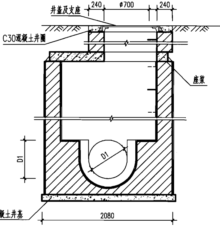
2-2 剖面
