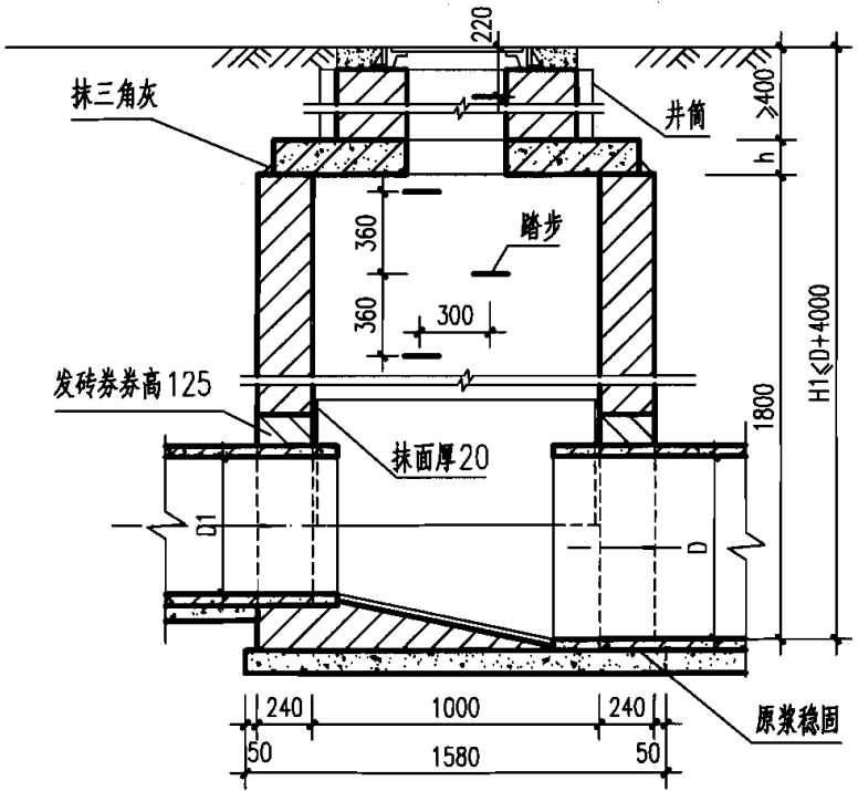
1-1 剖面
