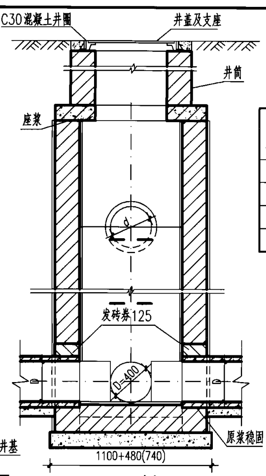
工程数量表 (按D=400计算)
