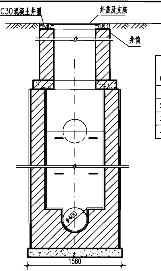
2-2 剖面
