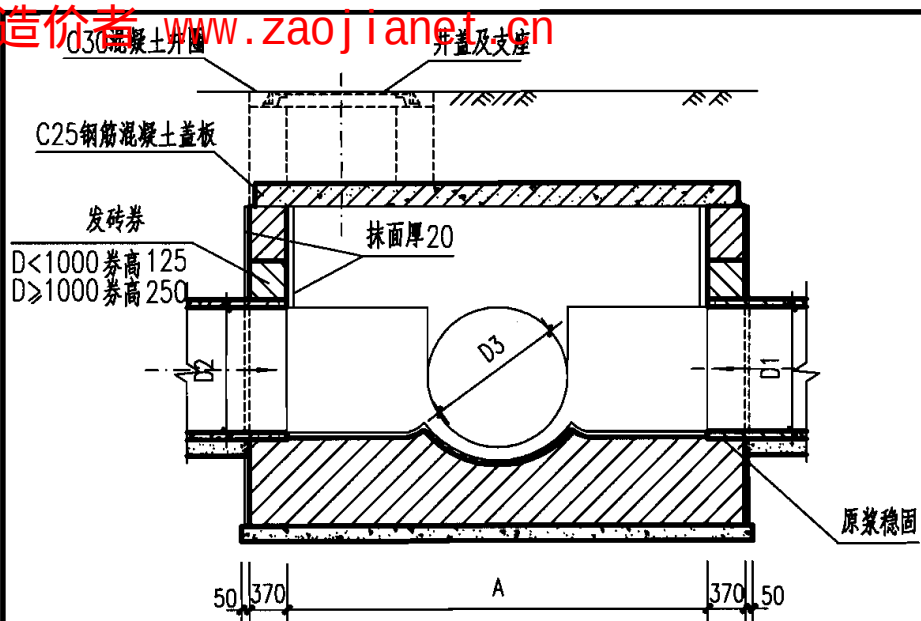
1-1 剖面
