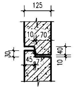
企口尺寸大样
