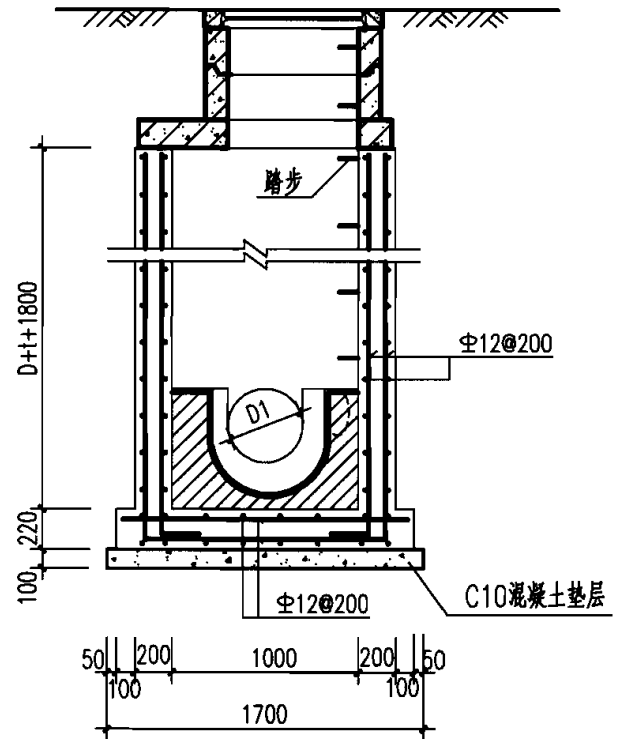
2-2 剖面
