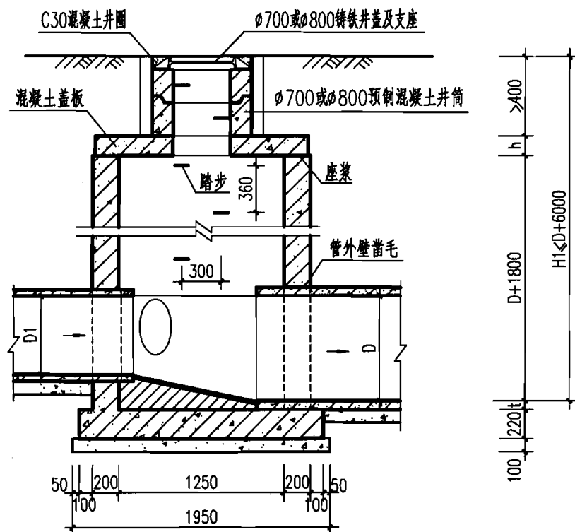
1-1 剖面
