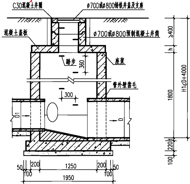
1-1 剖面
