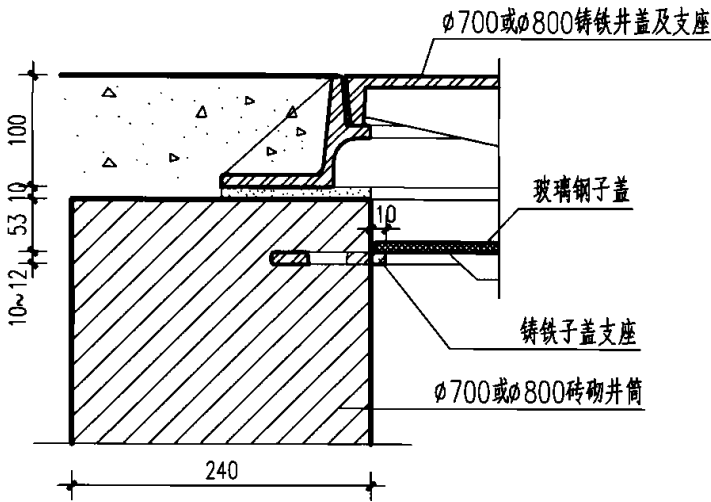
子盖安装大样图
