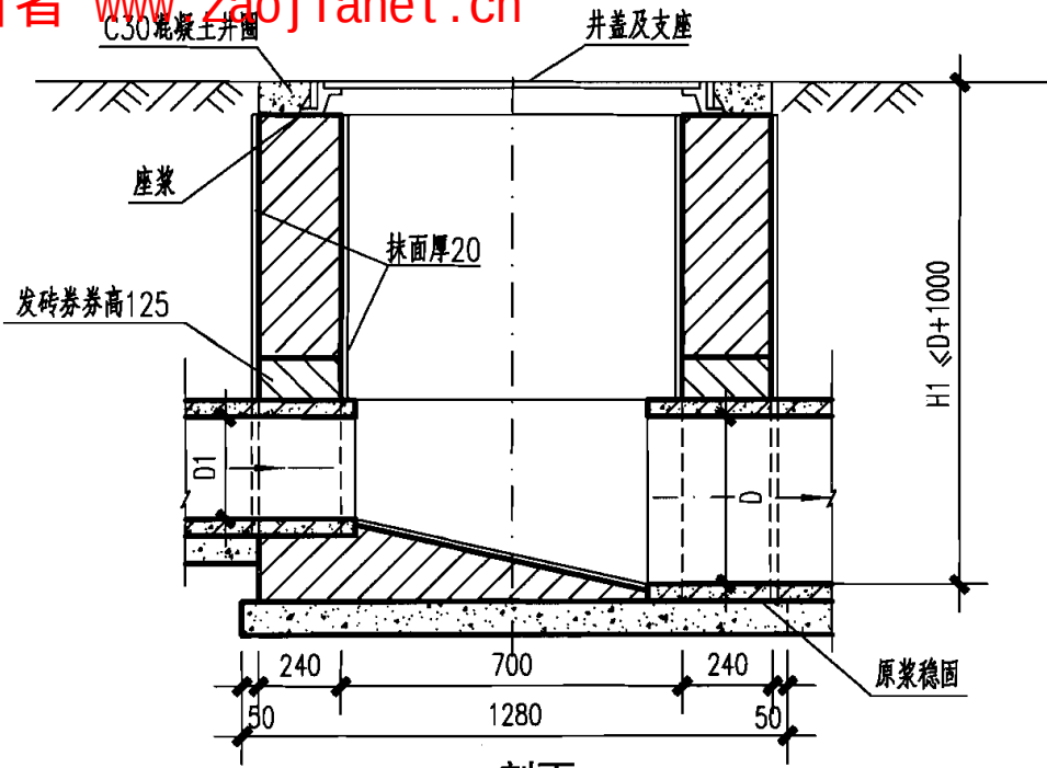
1-1 剖面
