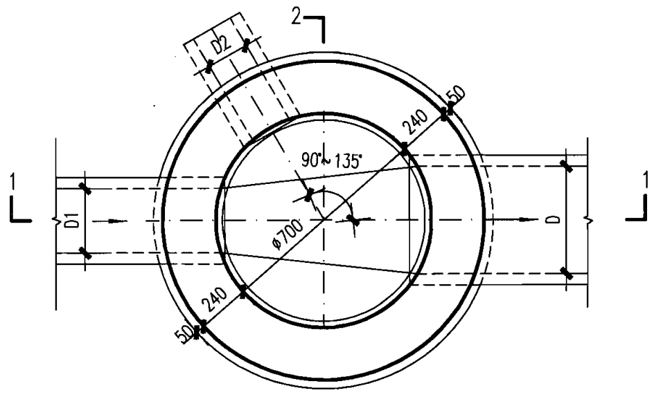
2 平面图
