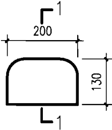
脚窝立面
