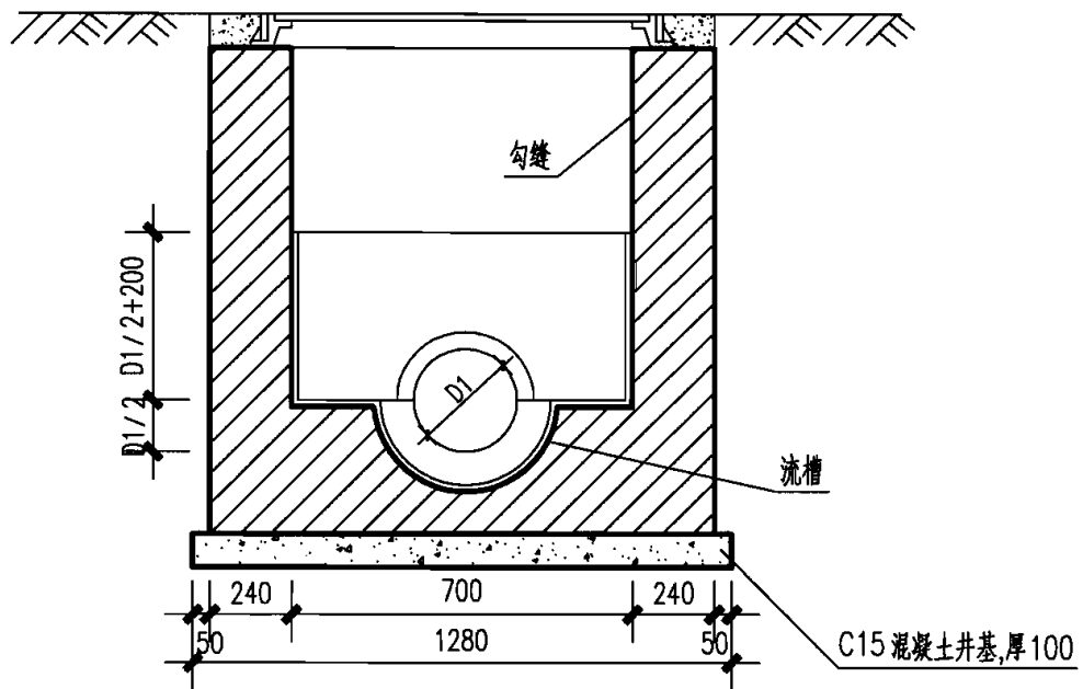
2-2 剖面
