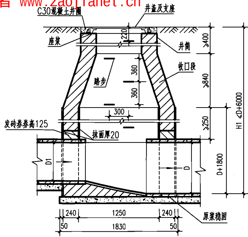
1-1 剖面
