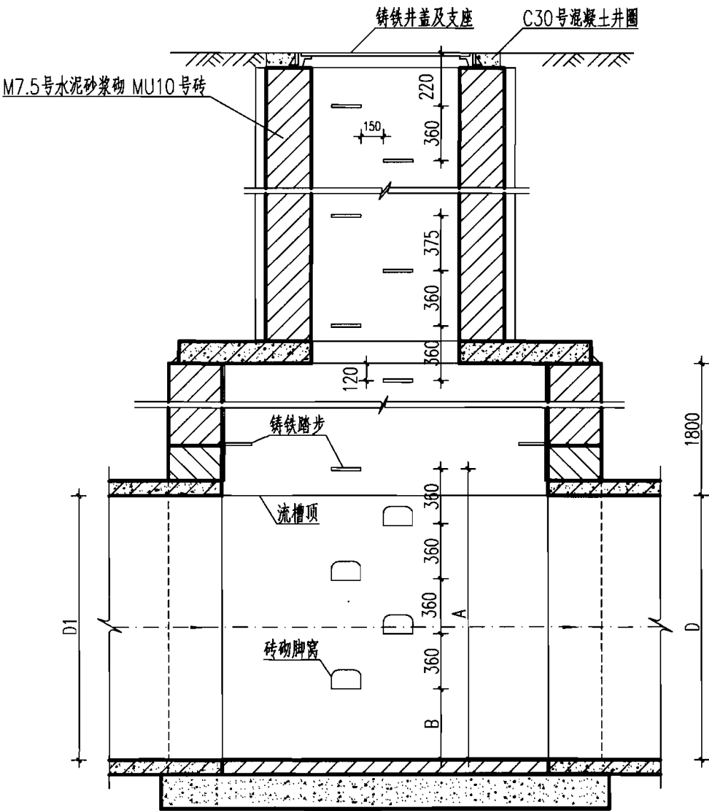
污水检查井剖面图
