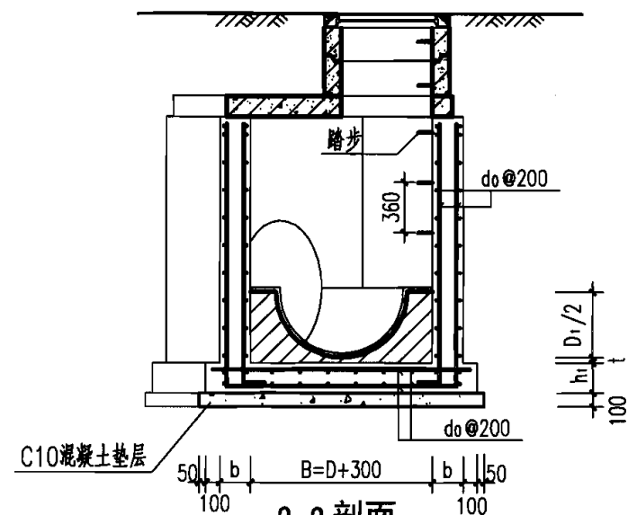
2-2 剖面
