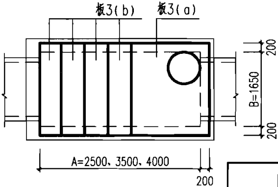
盖板布置图
