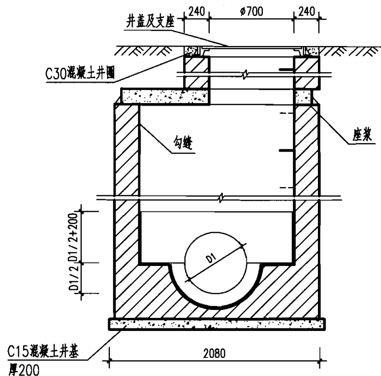
2-2 剖面
