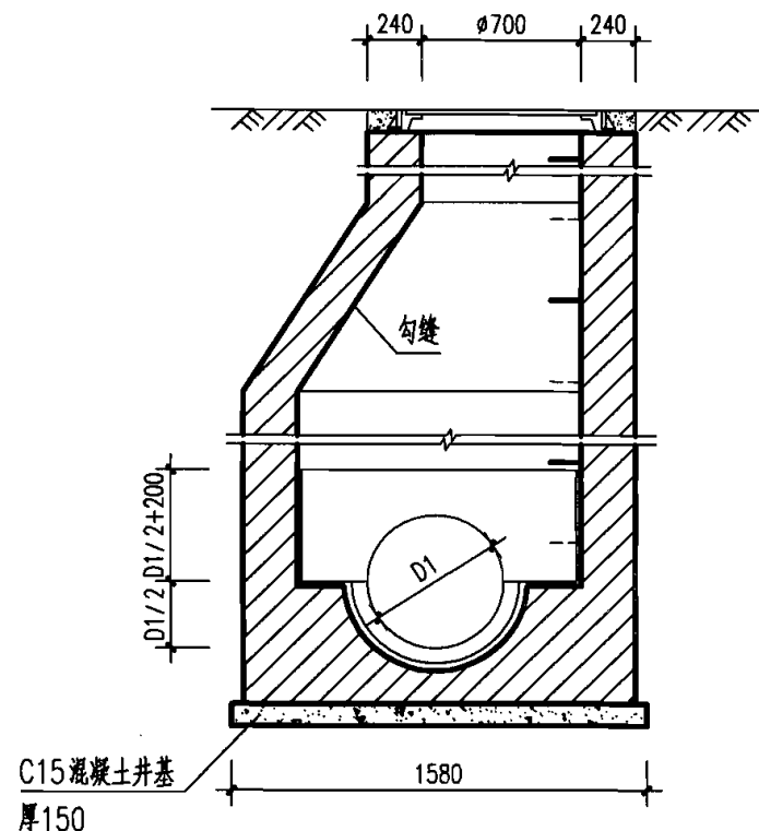
2-2 剖面
