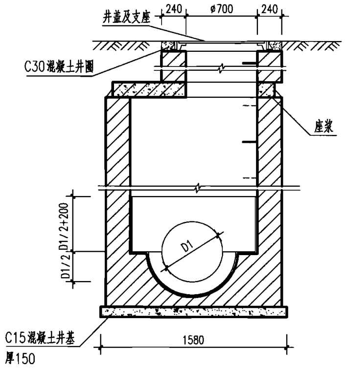
2-2 剖面
