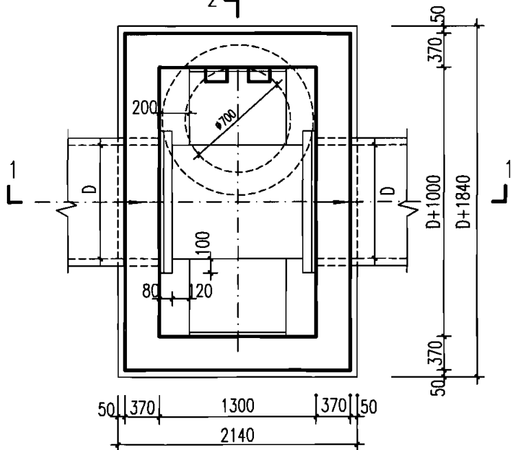
平面图
