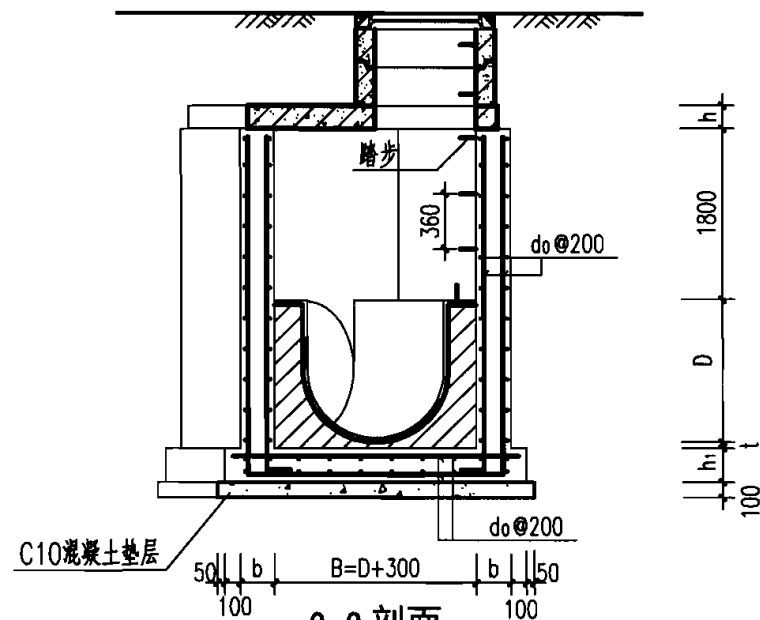
2-2 剖面
