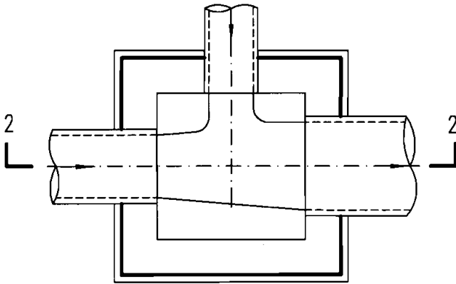
90°三通井平面图
