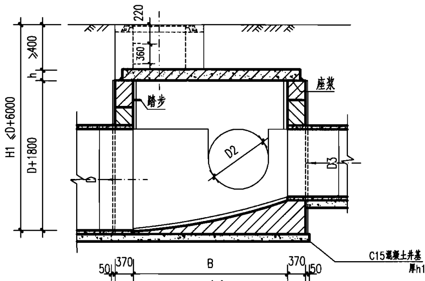
2-2 剖面
