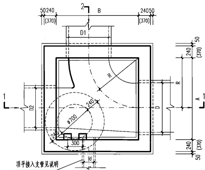
平面图
