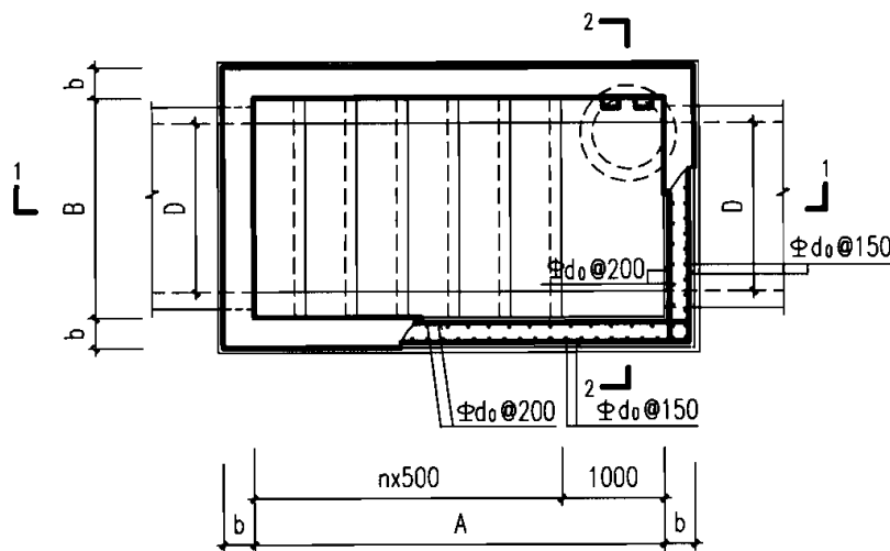
井室平面图 1:50
