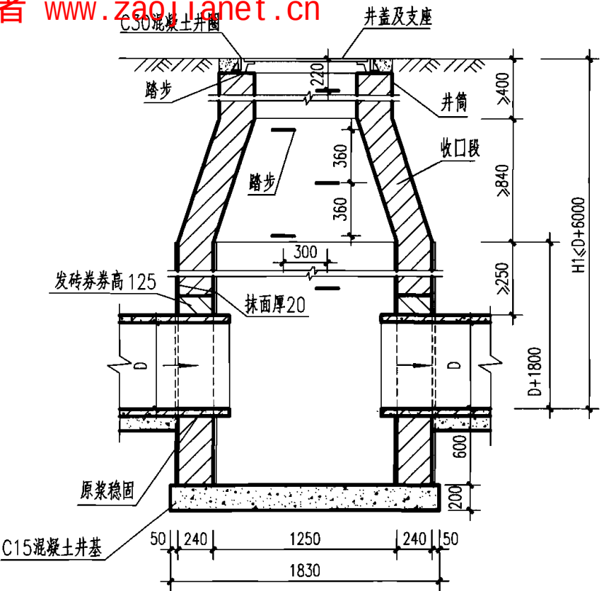
1-1 剖面
