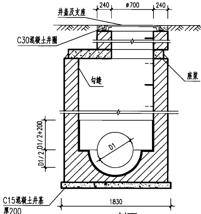
2-2 剖面
