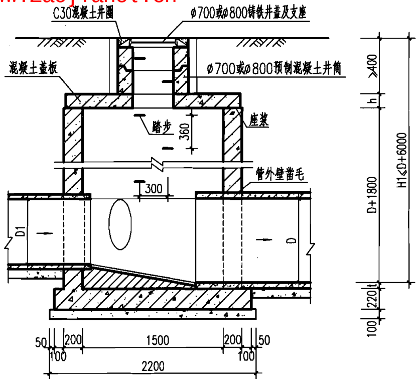
1-1 剖面
