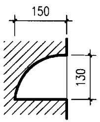
1-1剖面
