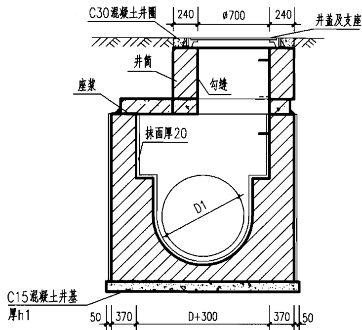
2-2 剖面
