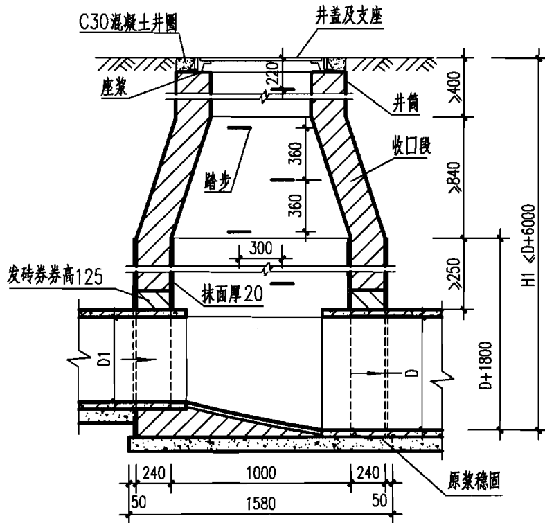
1-1 剖面
