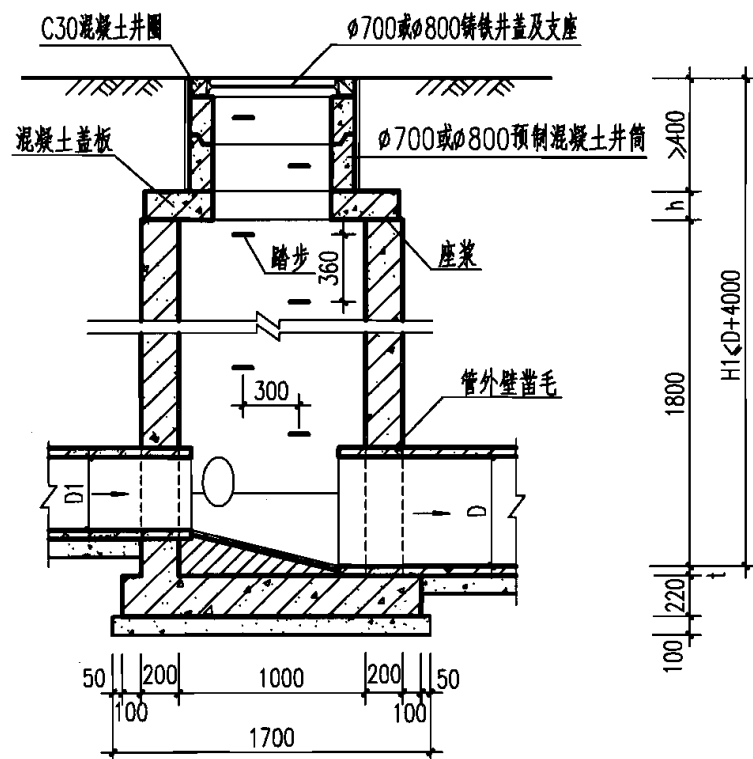
1-1 剖面
