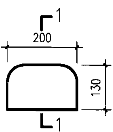
脚窝立面
