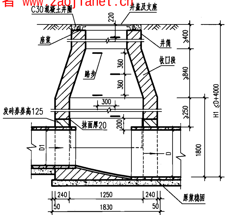
1-1 剖面
