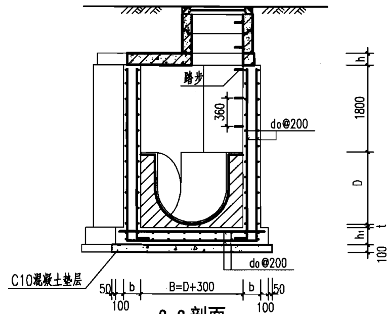
2-2 剖面
