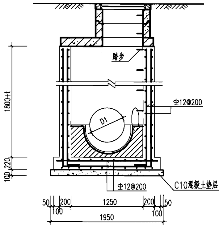
2-2 剖面
