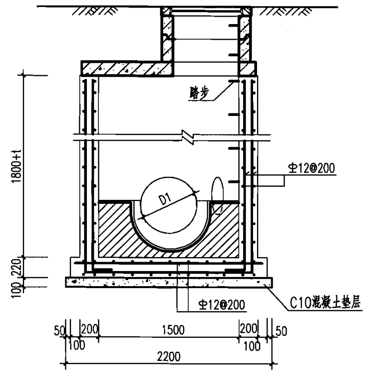
2-2 剖面
