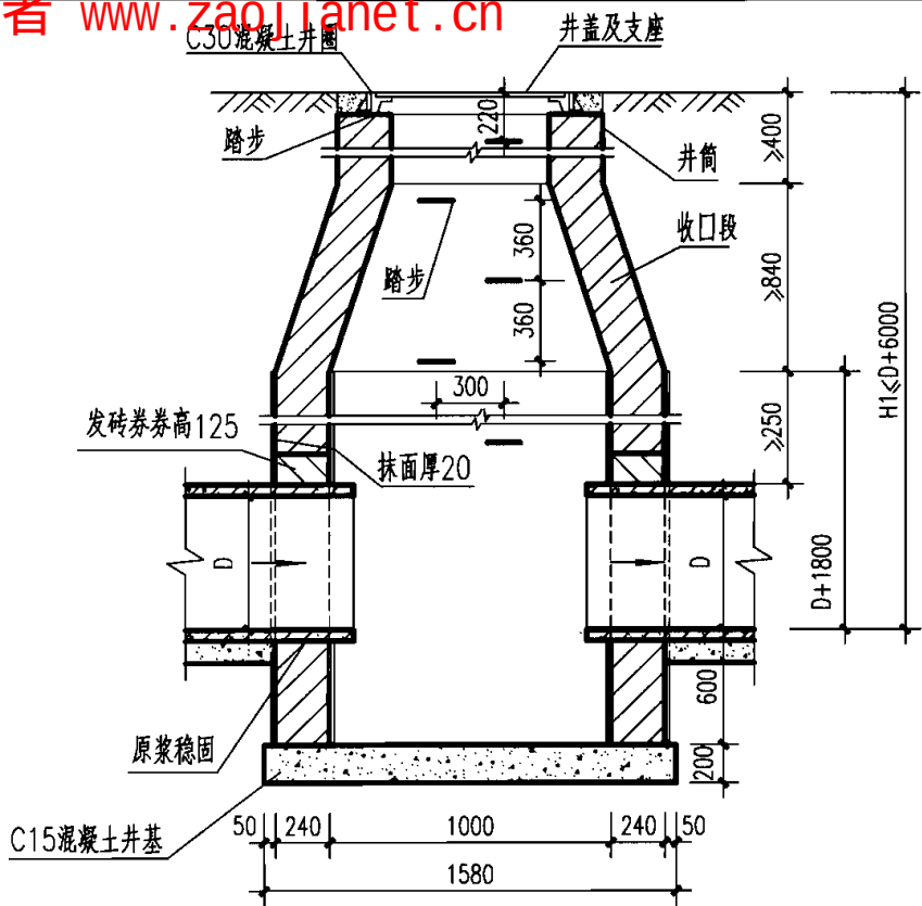
1-1 剖面
