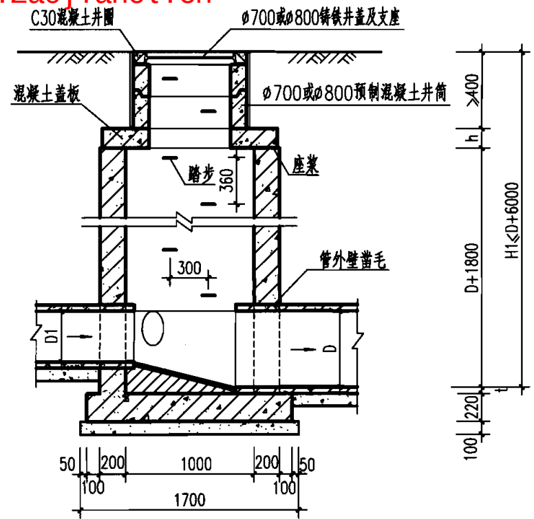
1-1 剖面
