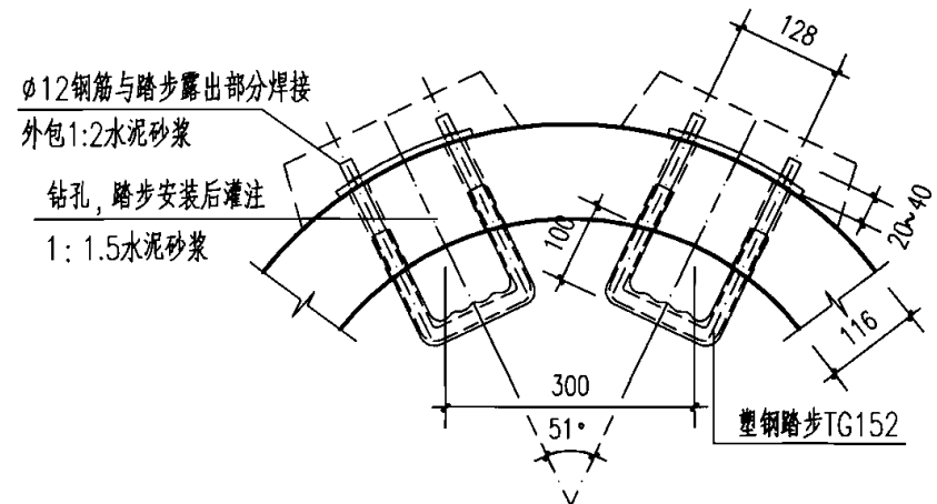
塑钢踏步安装大样
