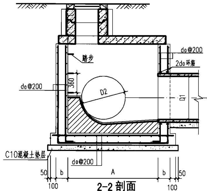
井室尺寸及配筋表
