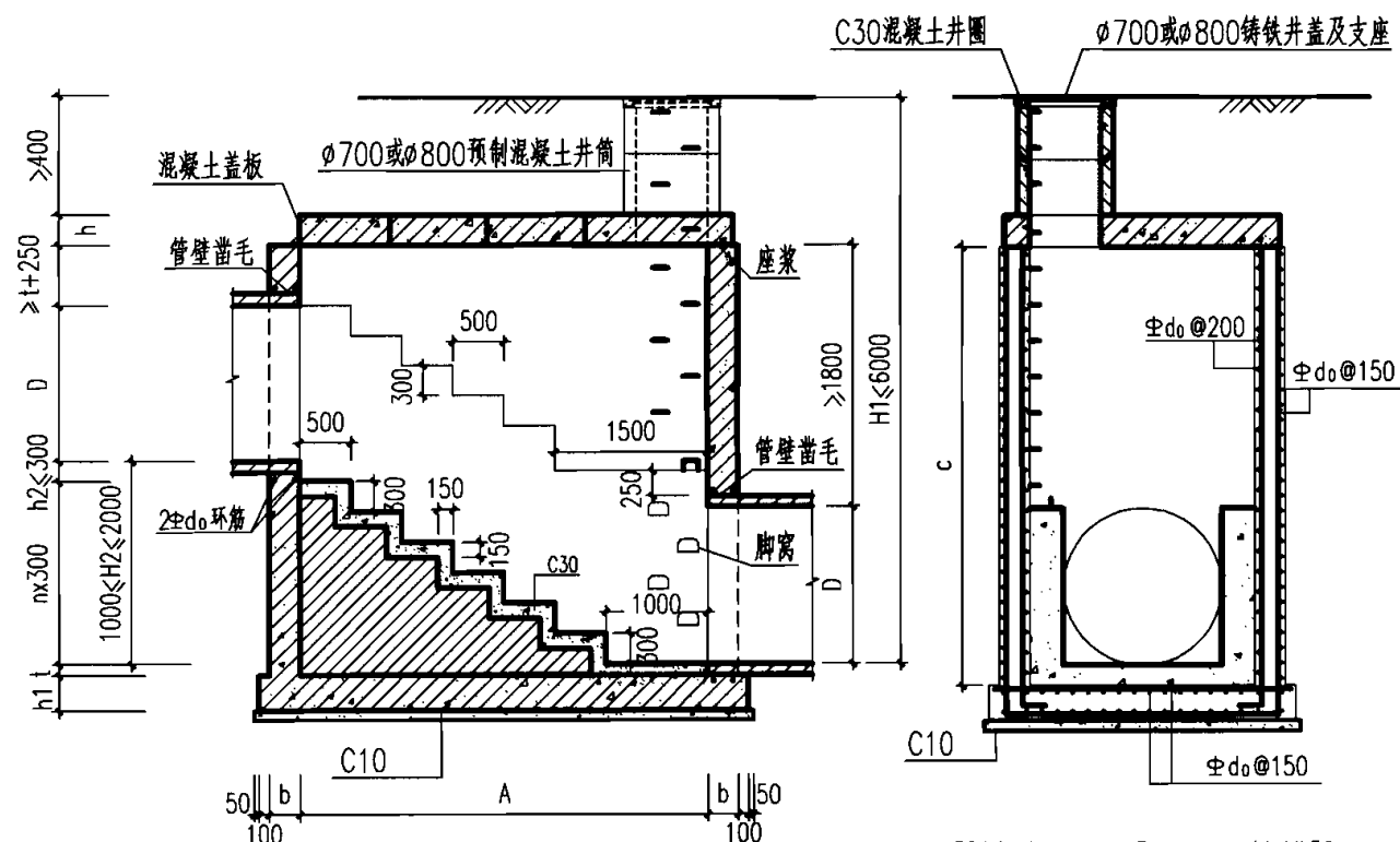
1-1 剖面 1:50
