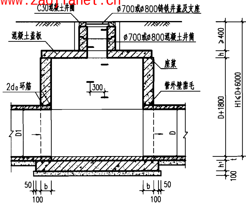
1-1 剖面
