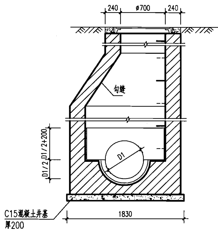
2-2 剖面
