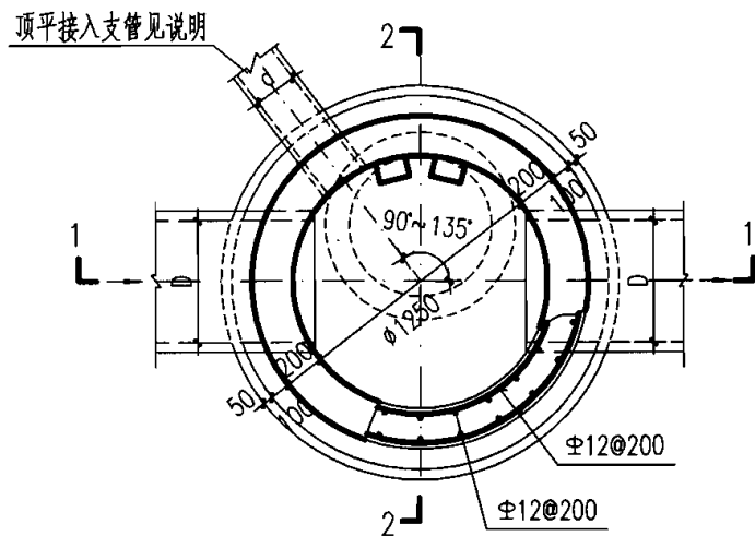
平面图
