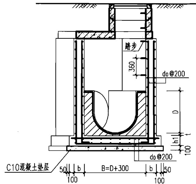
2-2 剖面
