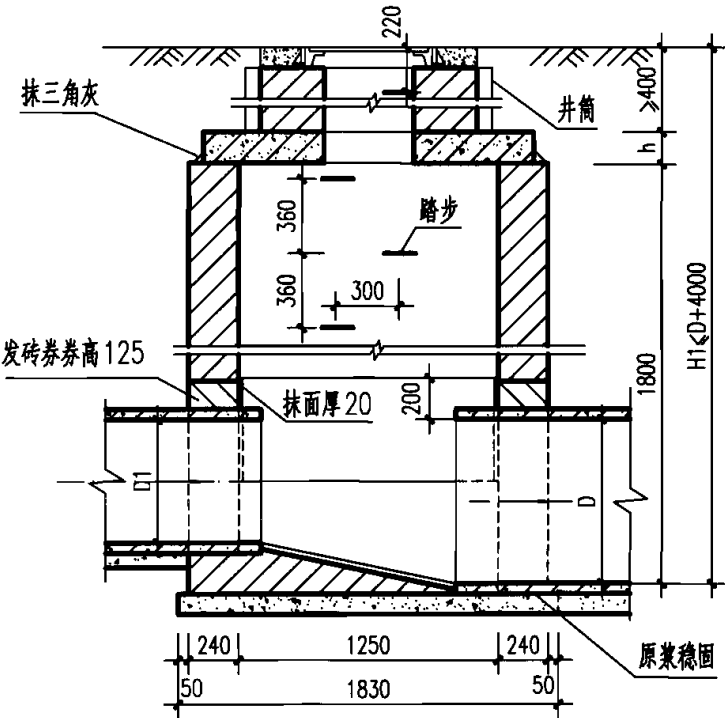
1-1 剖面
