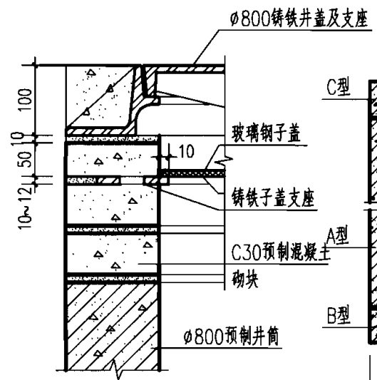
子盖安装大样
