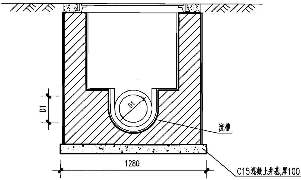
2-2 剖面
