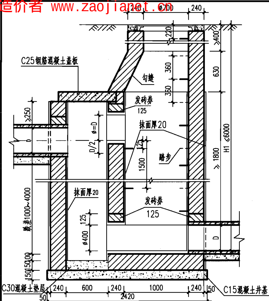
1-1 剖面
