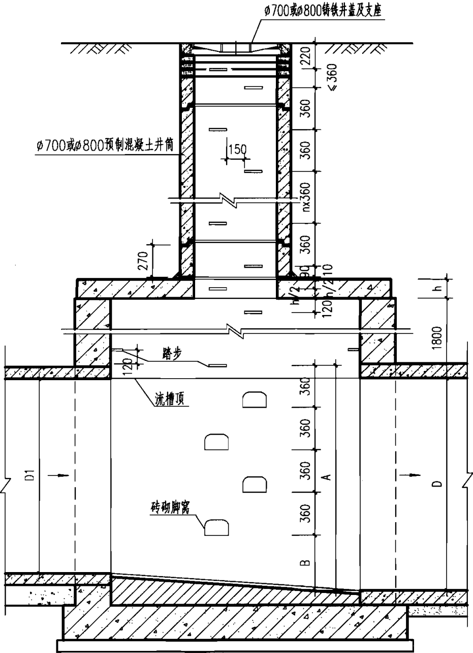
污水检查井剖面图
