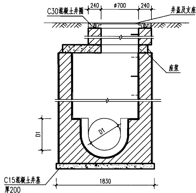
2-2 剖面
