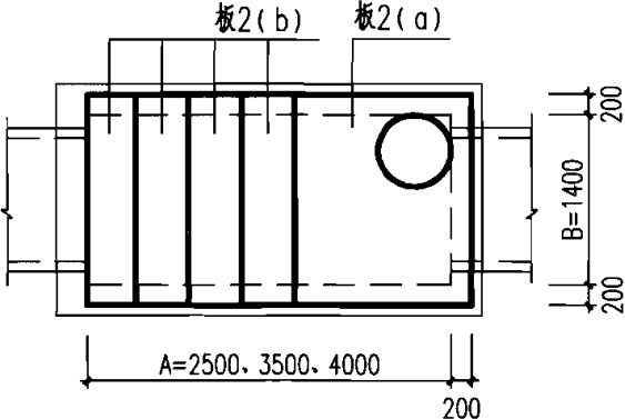
盖板布置图
