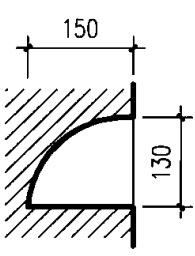
1-1剖面
