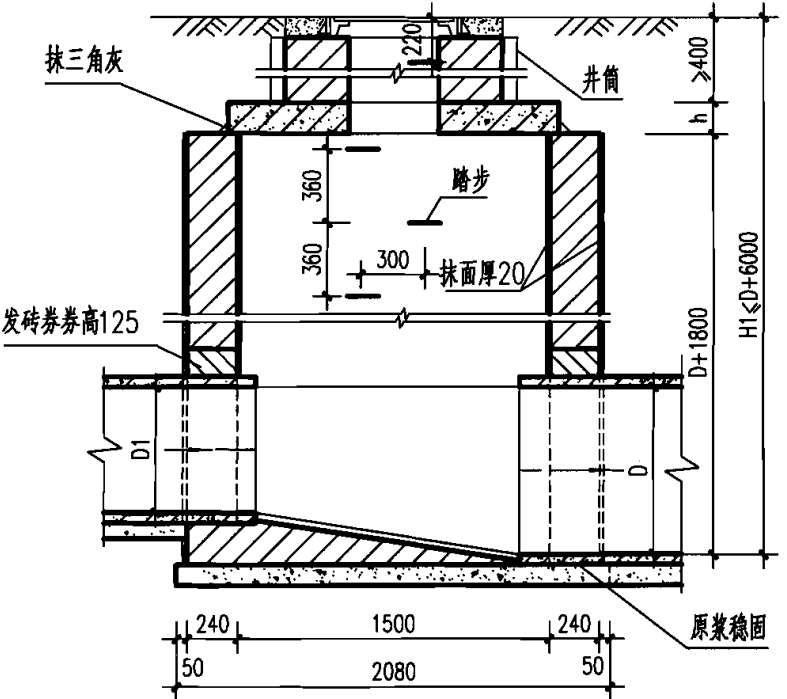
1-1 剖面
