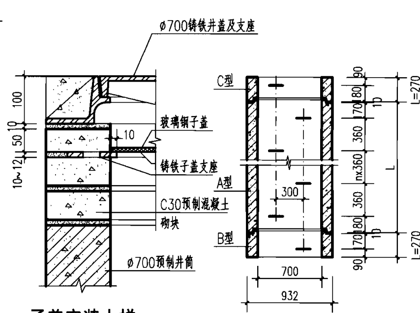
子盖安装大样
