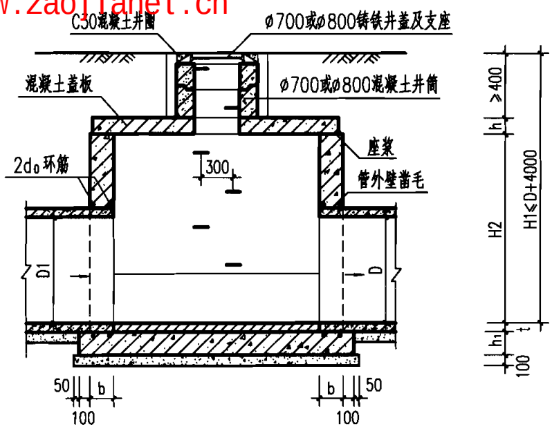
1-1 剖面
