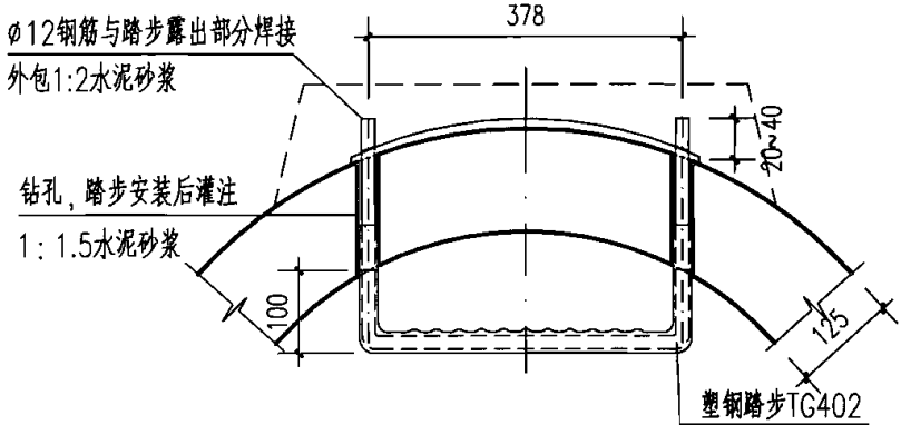
塑钢踏步安装大样
