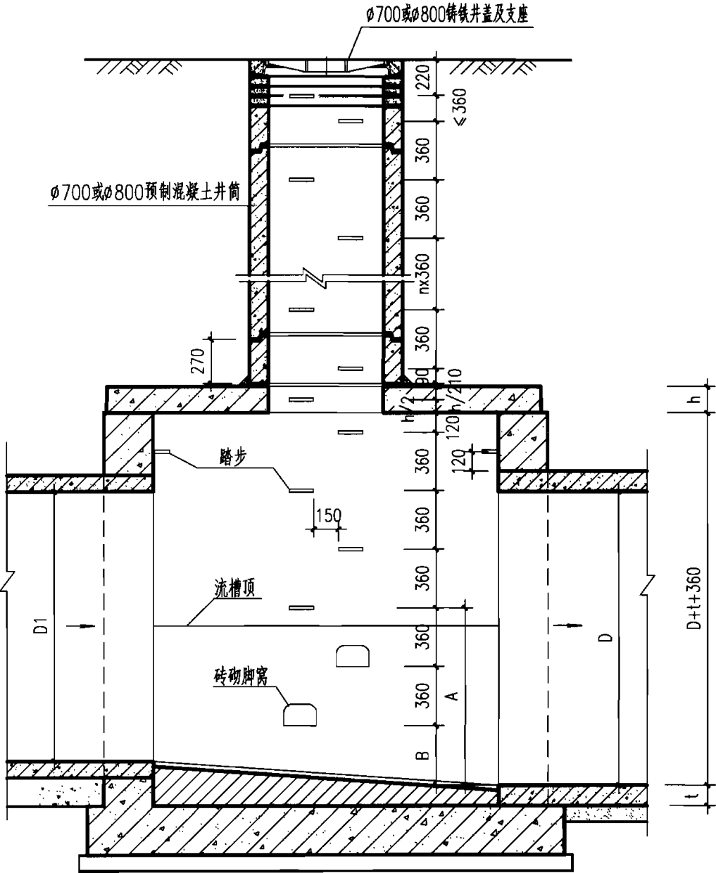
雨水检查井剖面图
