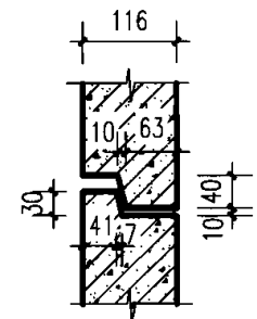
企口尺寸大样
