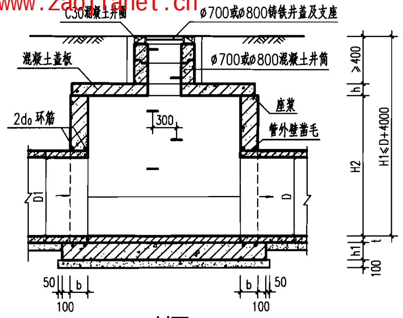
1-1 剖面
