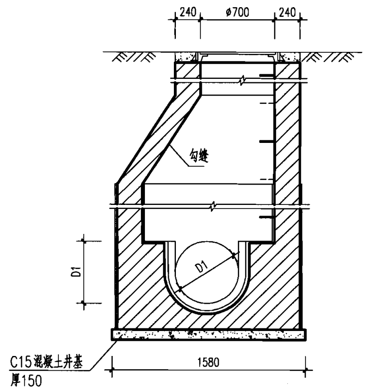
2-2 剖面
