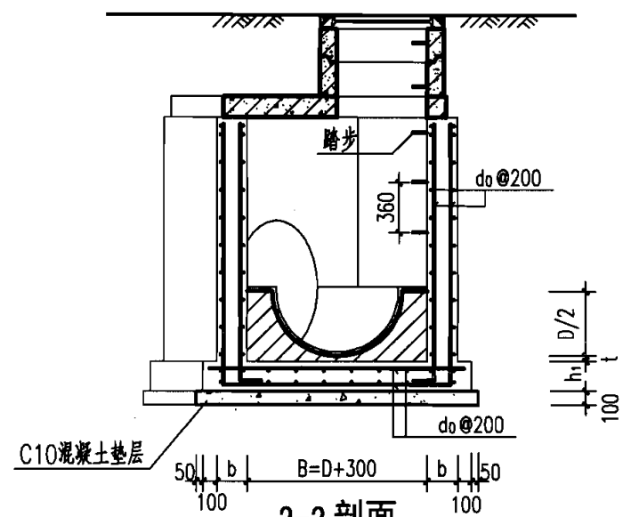
2-2 剖面
