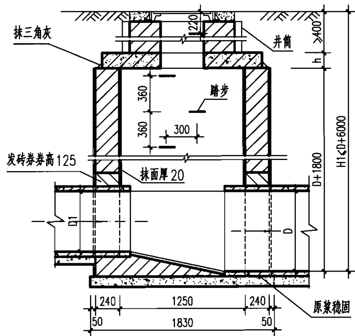
1-1 剖面
