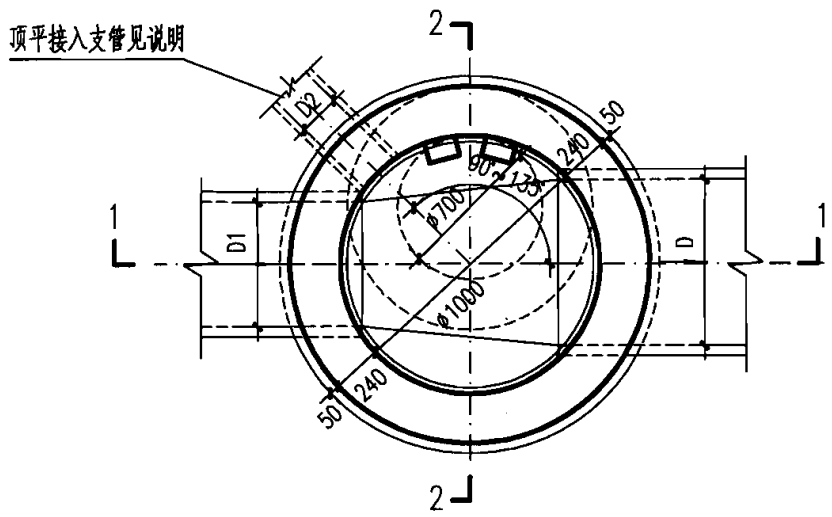
平面图
