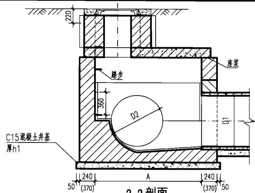
2-2 剖面
