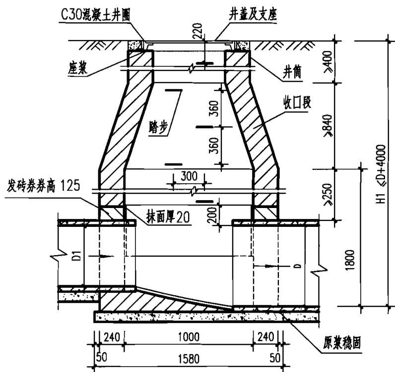
1-1 剖面
