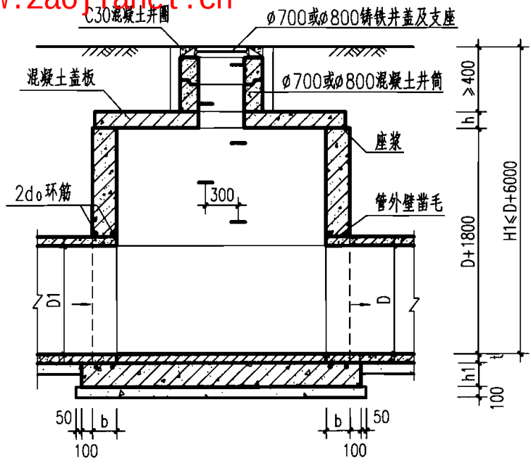
1-1 剖面
