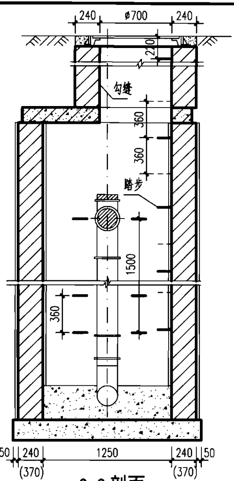
2-2 剖面
