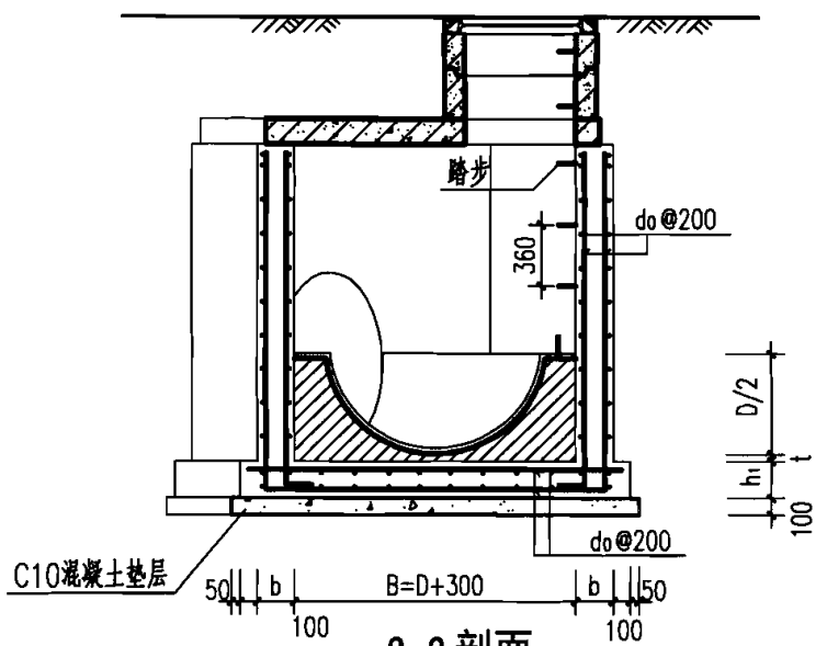
2-2 剖面
