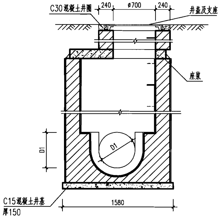
2-2 剖面
