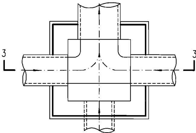
90°四通井平面图
