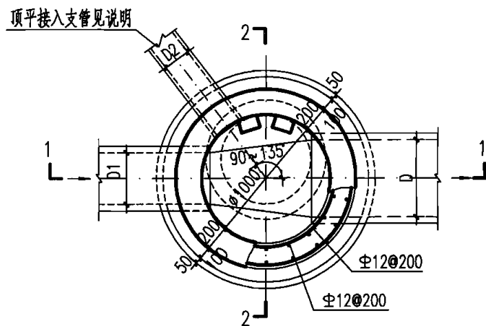
平面图
