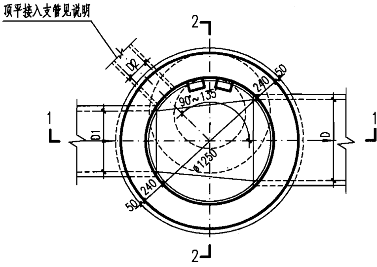
2 平面图
