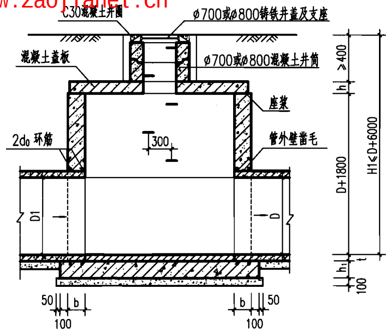
1-1 剖面
