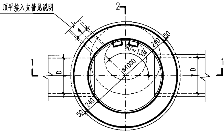
2-2 剖面
