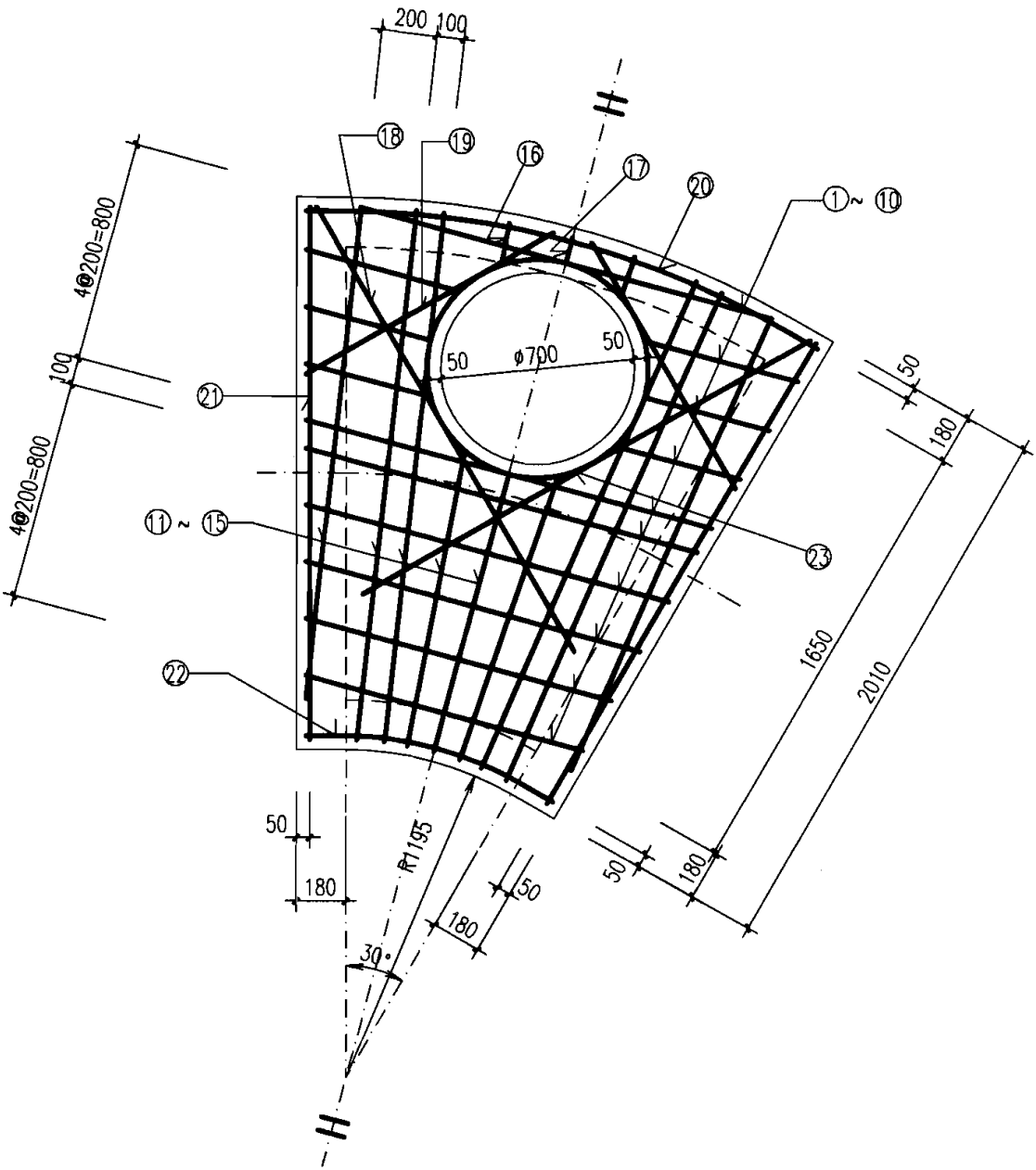
扇形雨污水检查井 ( 150° ) 盖板配筋图 ③ (D=1200~1350)
