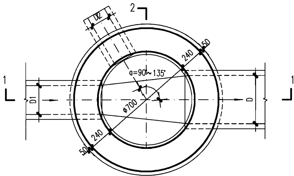
平面图
