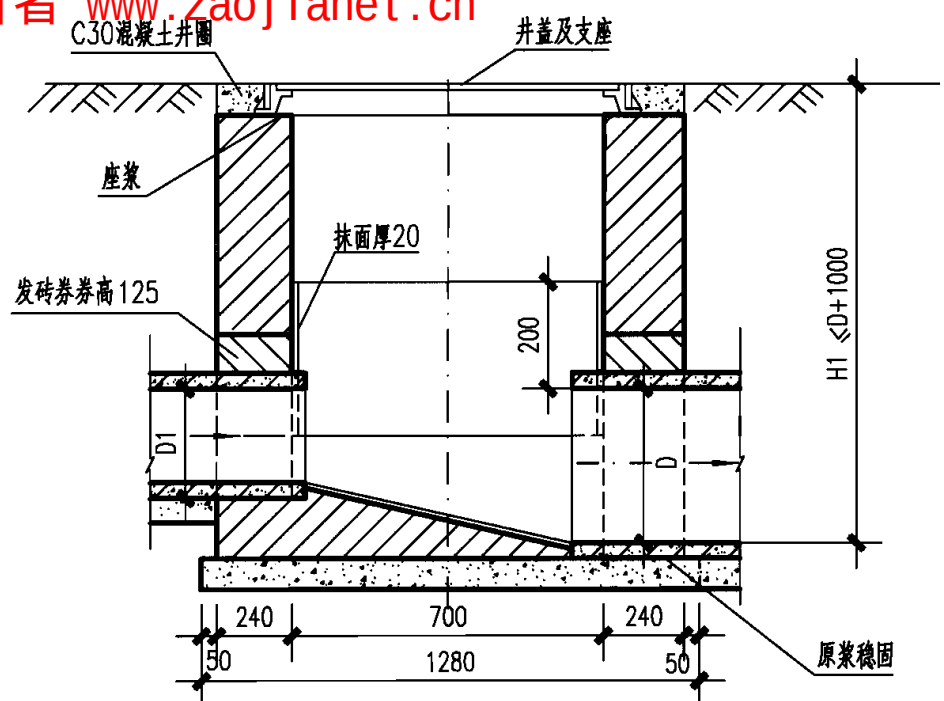
1-1 剖面
