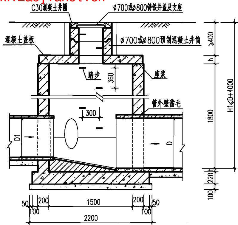
1-1 剖面
