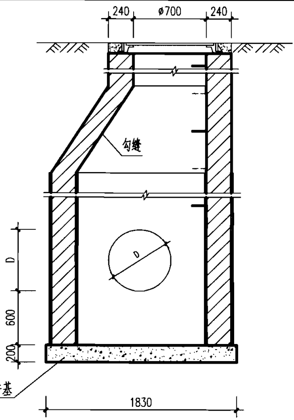
2-2 剖面
