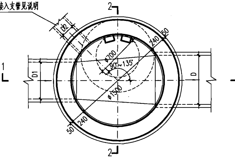
2 平面图
