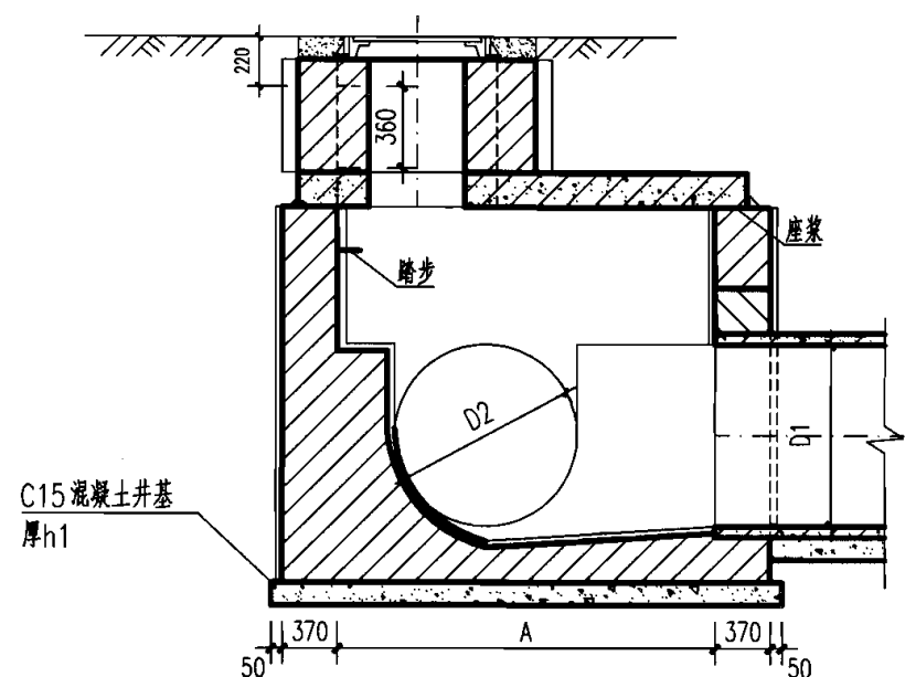
2-2 剖面
