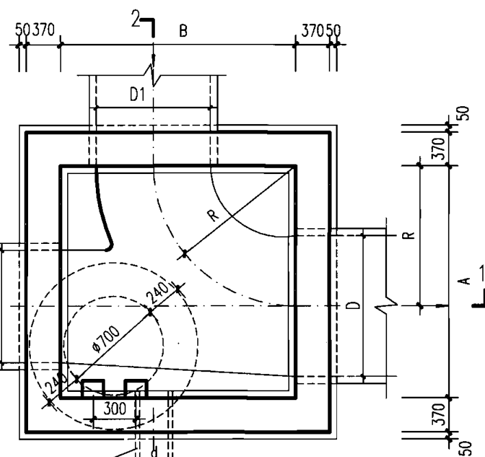
平面图
