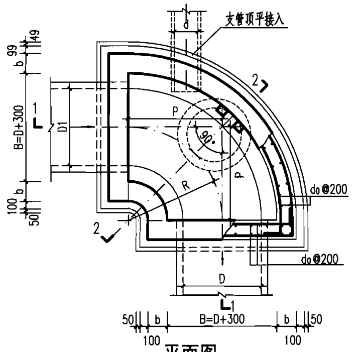
平面图
