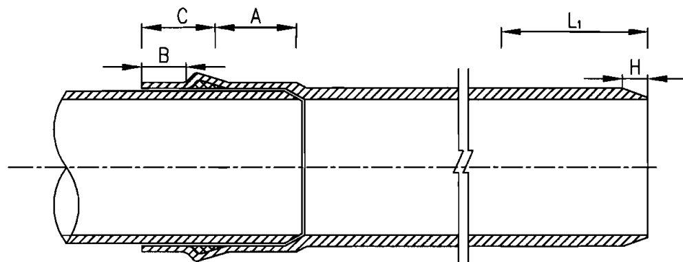
橡胶圈接口
