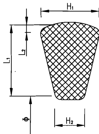
橡胶圈截面图
