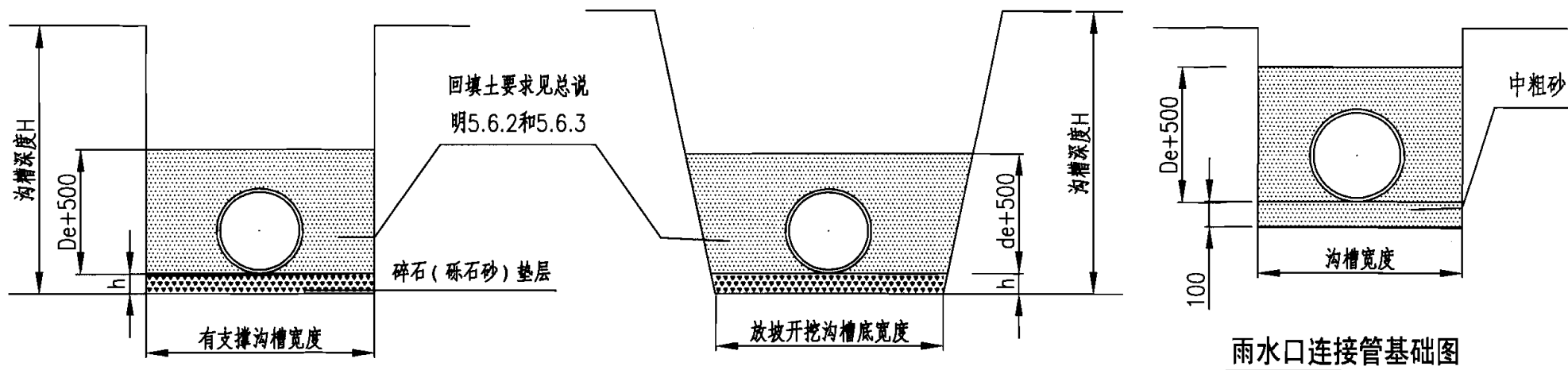
管道基础图
