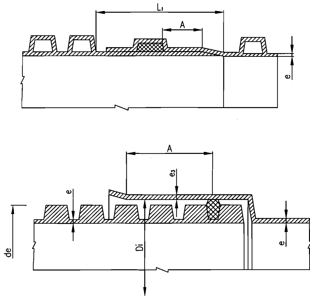
管材承插口
