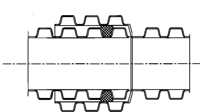
管道接口图
