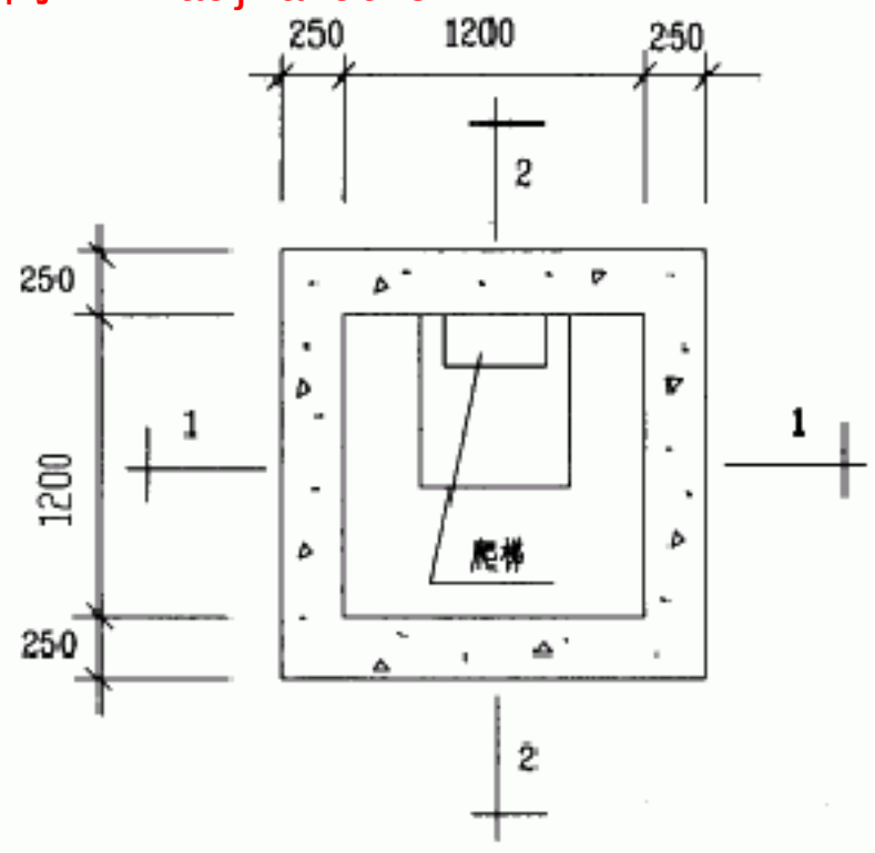
甲型平面
