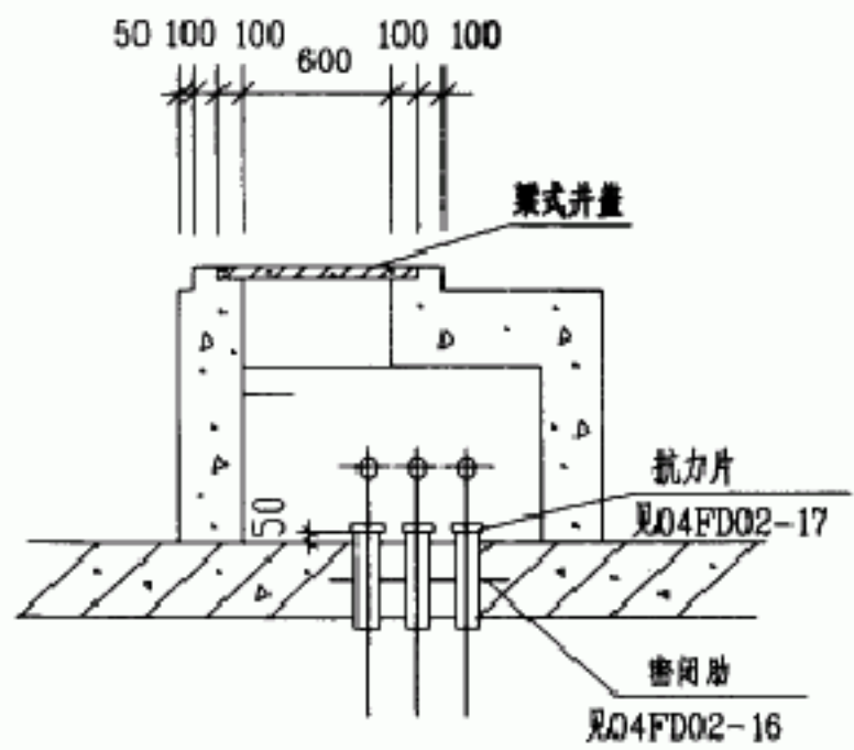
甲型2-2断面
