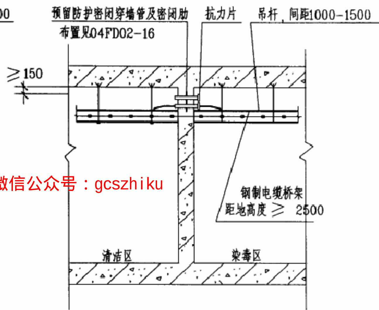
电缆桥架穿越人防围护墙做法(二)
