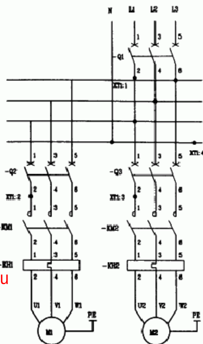
主回路
