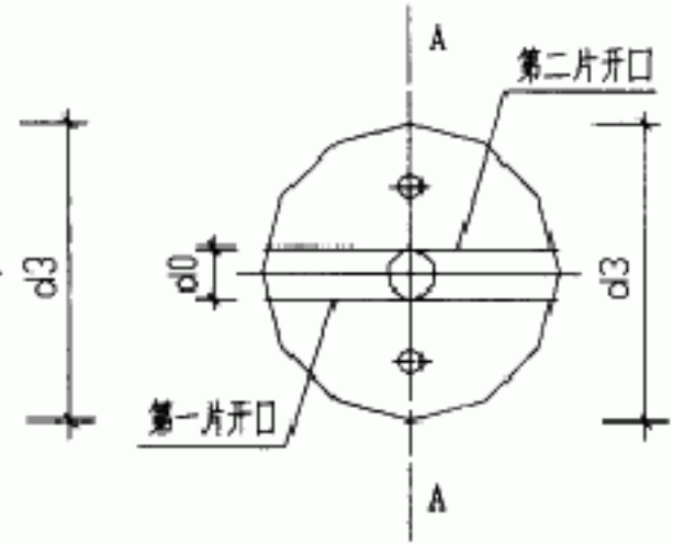
抗力片制作图
