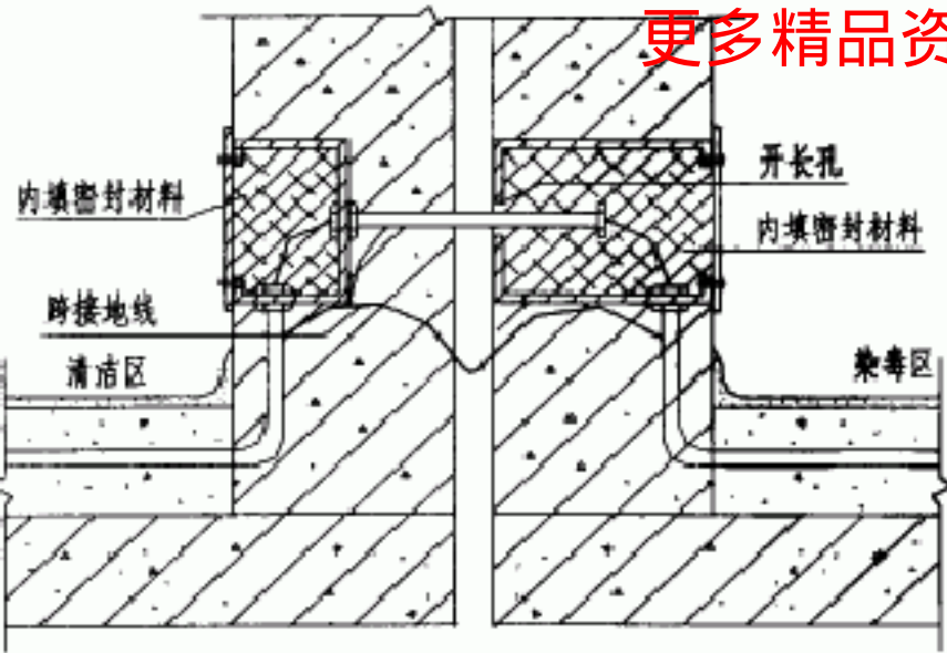
F 伸缩 沉降 缝接线盒做法
