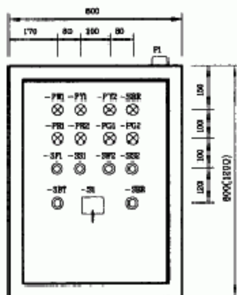
图面设备布置图
