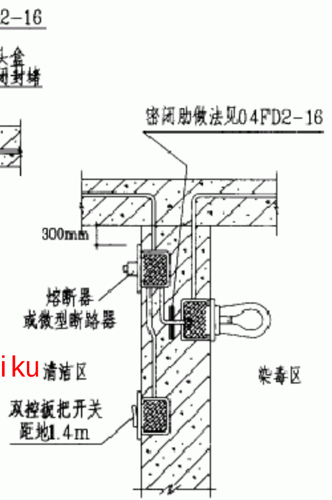
C 人防连通口照明灯具安装纵剖视图
