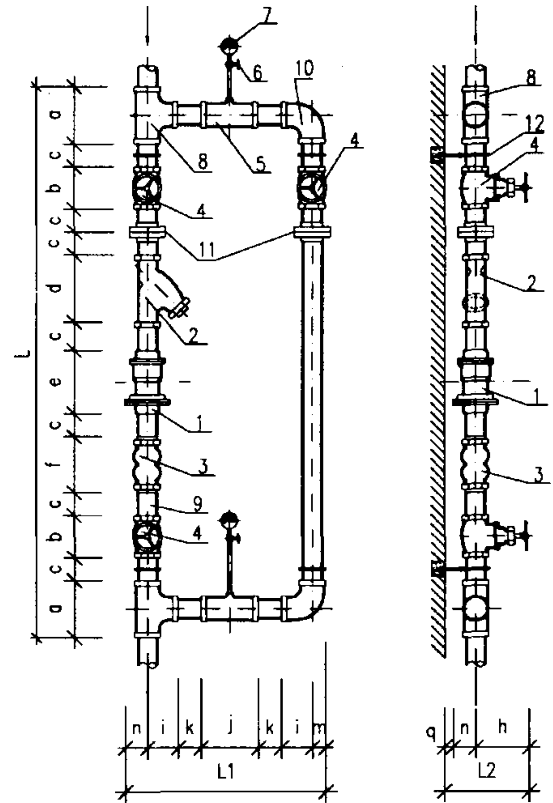
正视图
