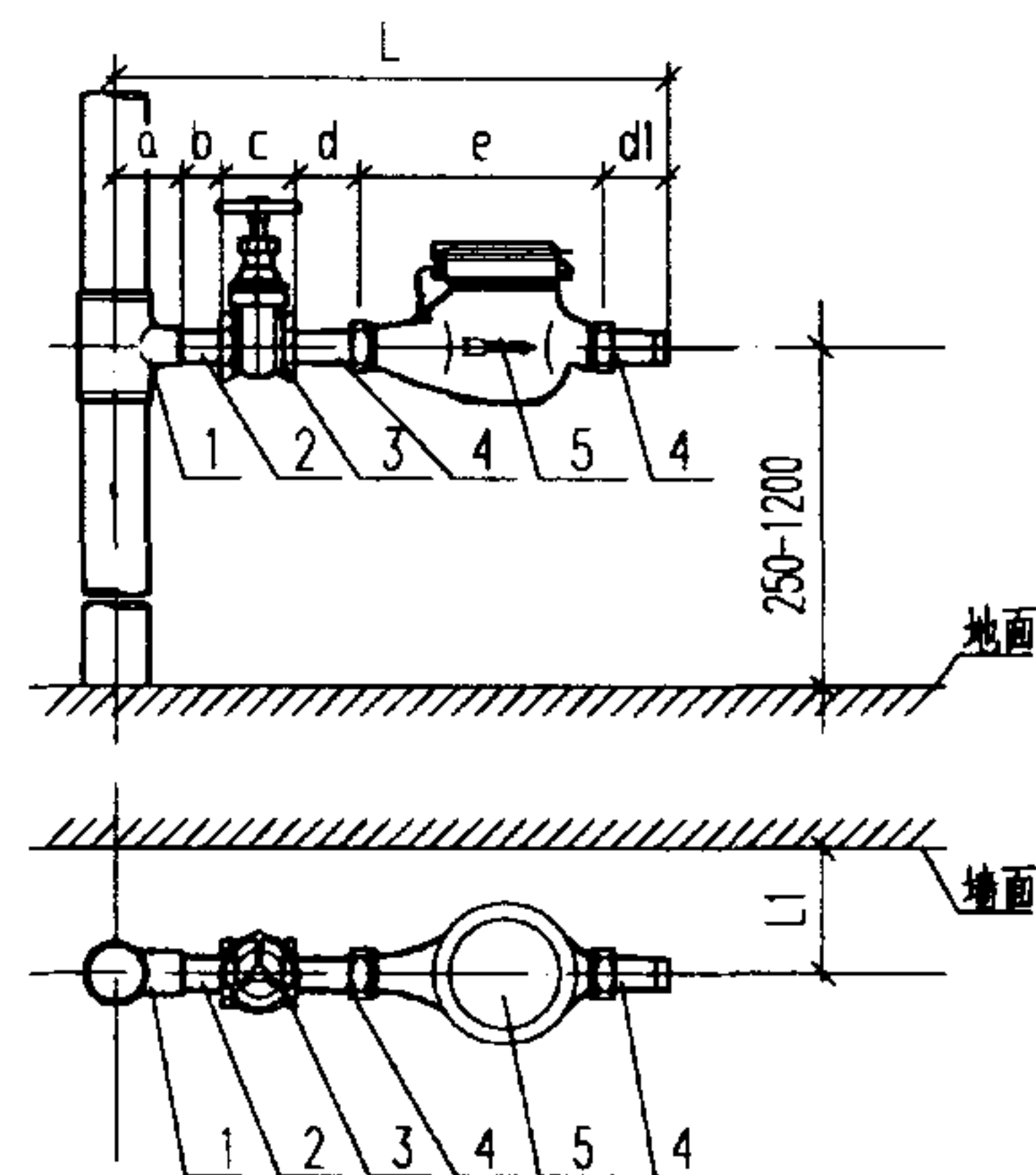
丙型安装图
