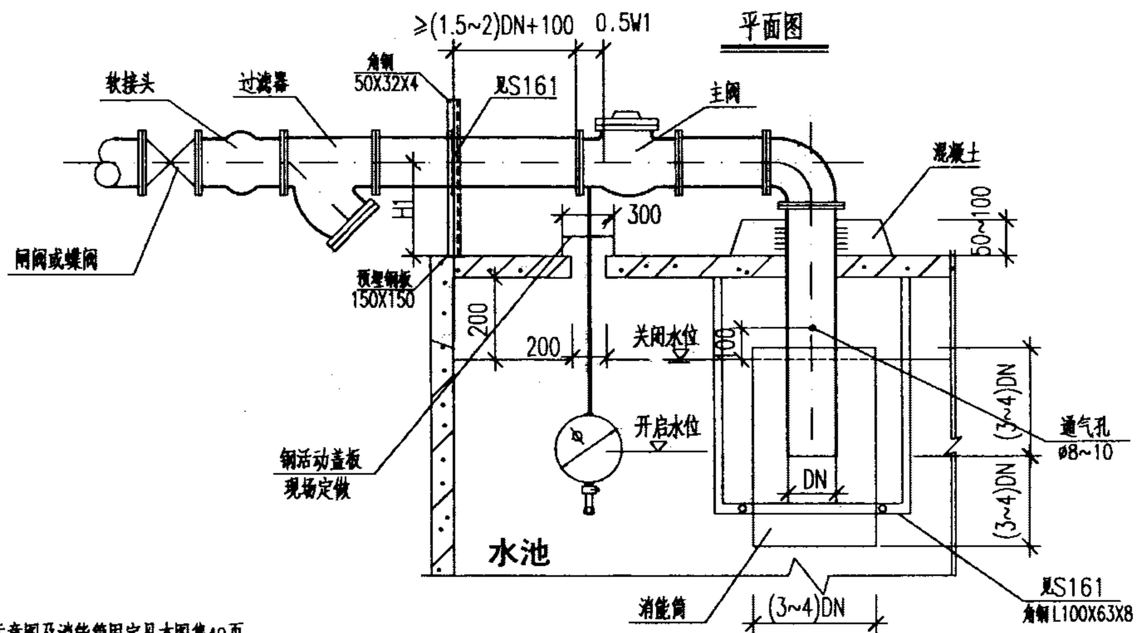
1-1 剖面图
