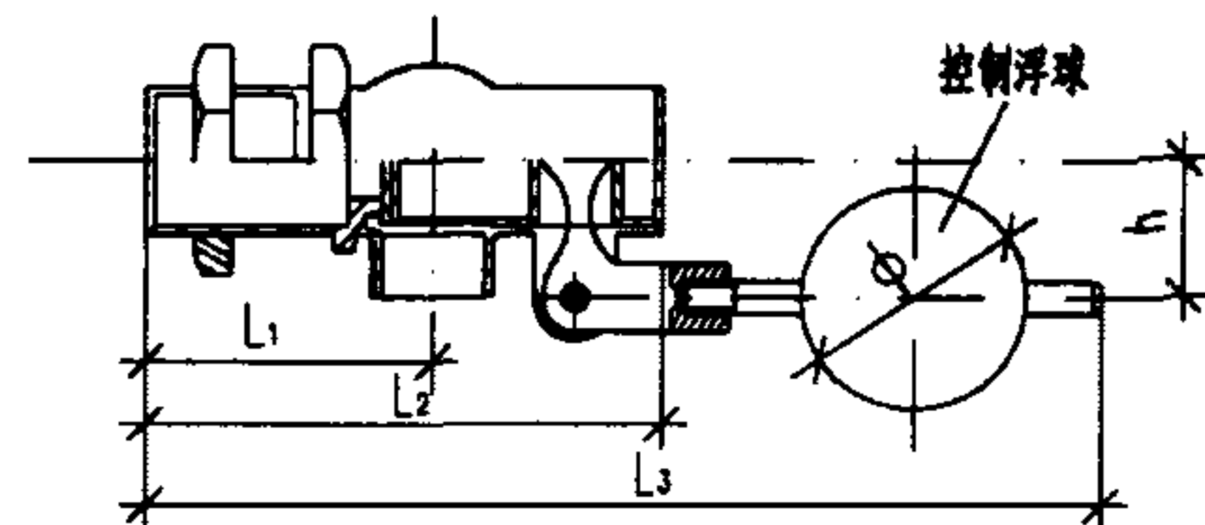
结构示意图
