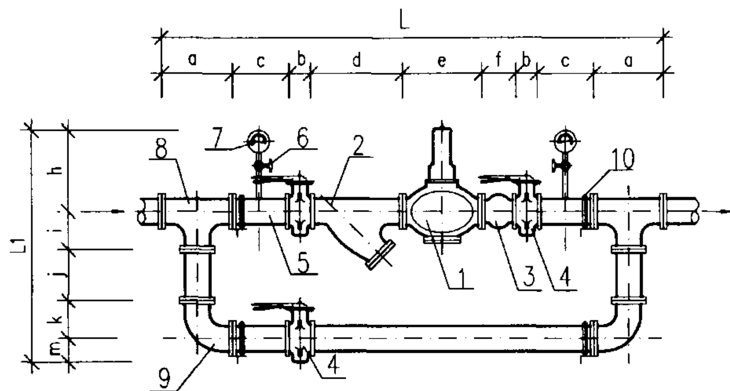
正视图
