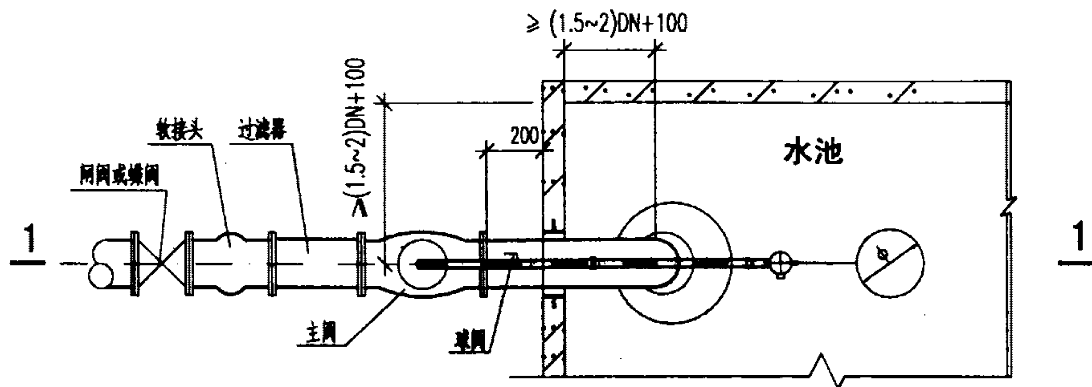
平面图
