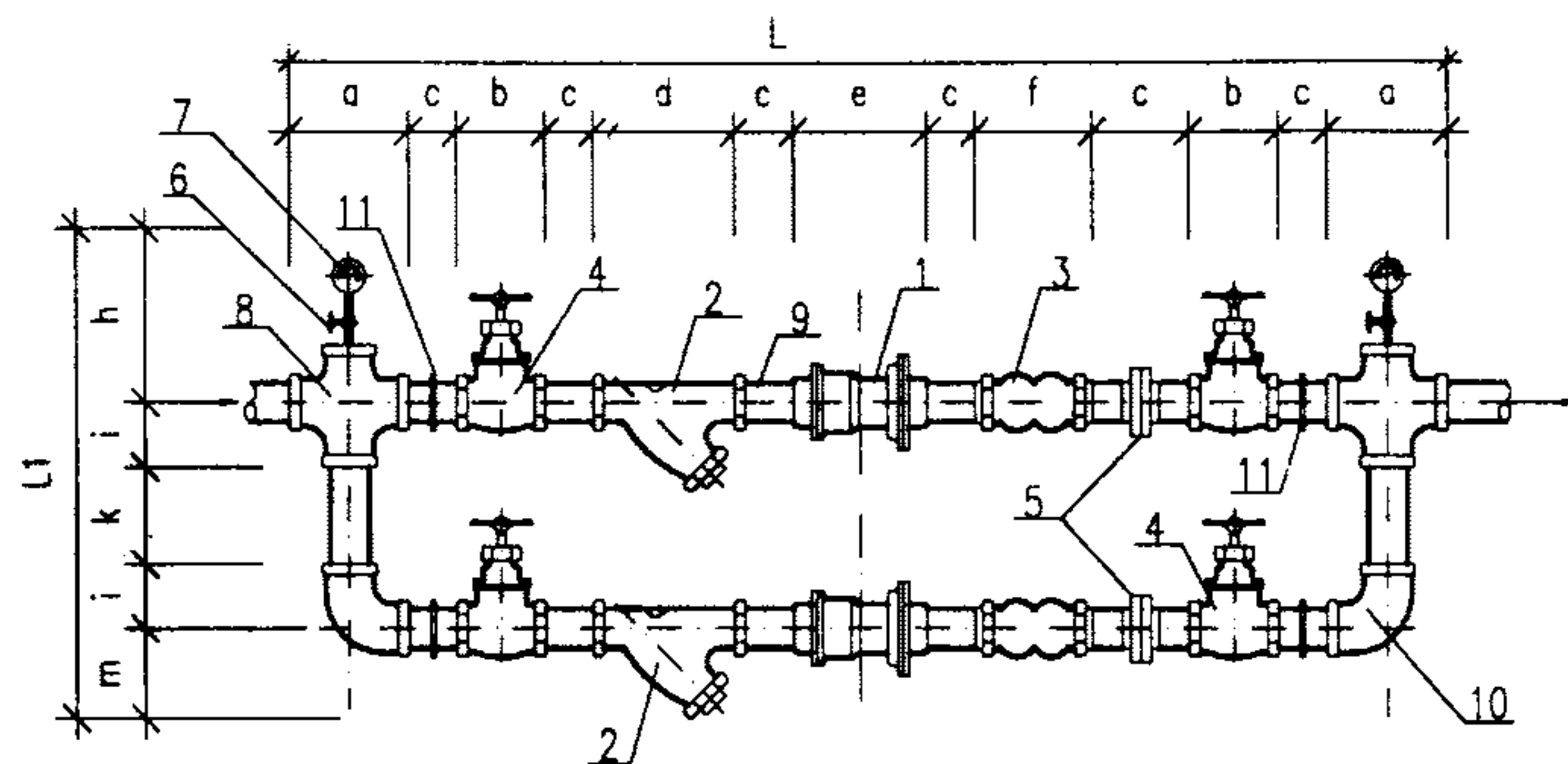
正视图
