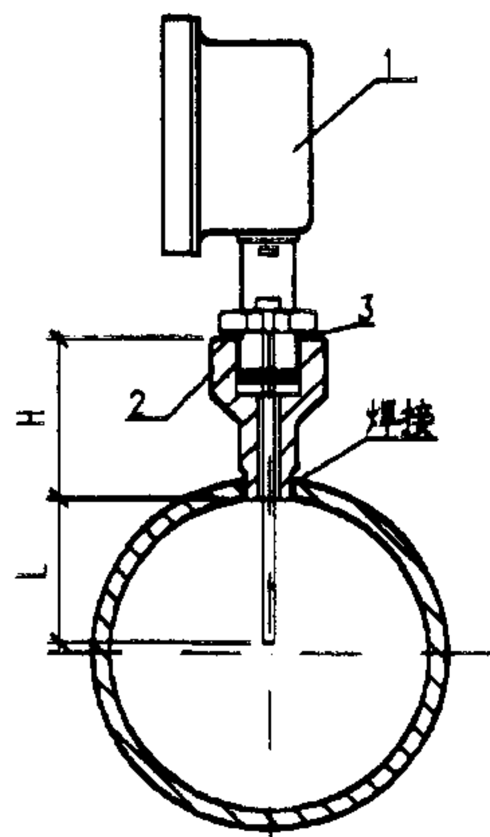
乙型
