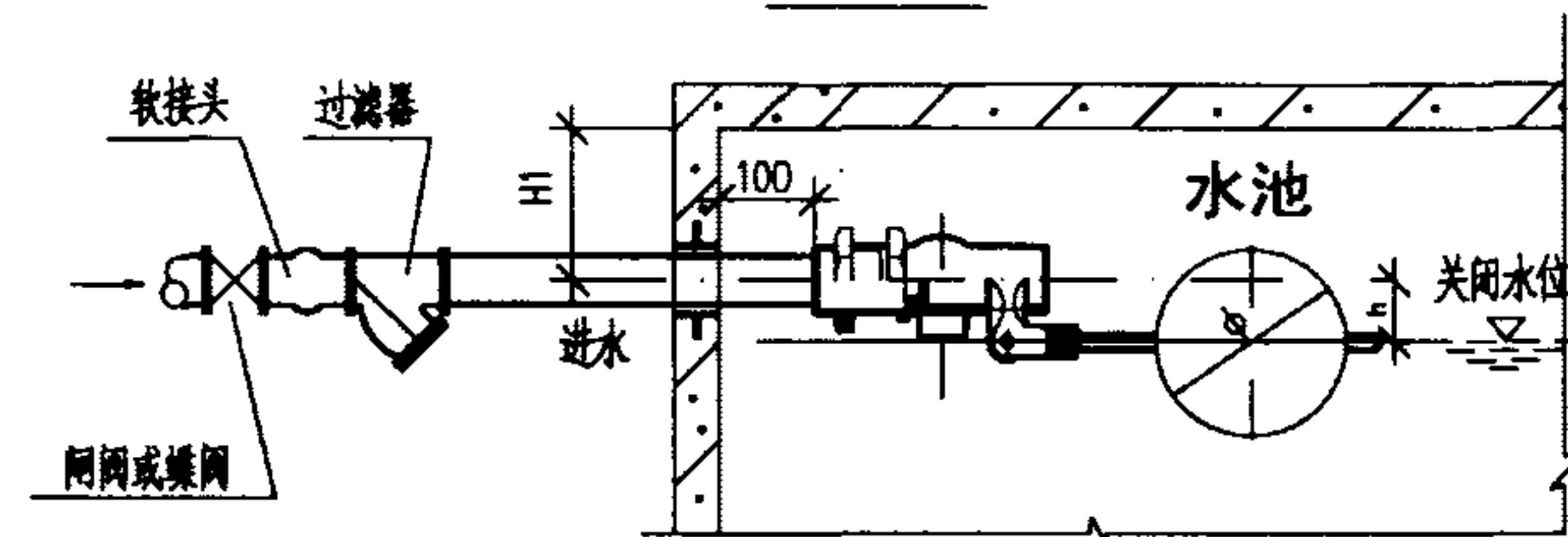
1-1 剖面图
