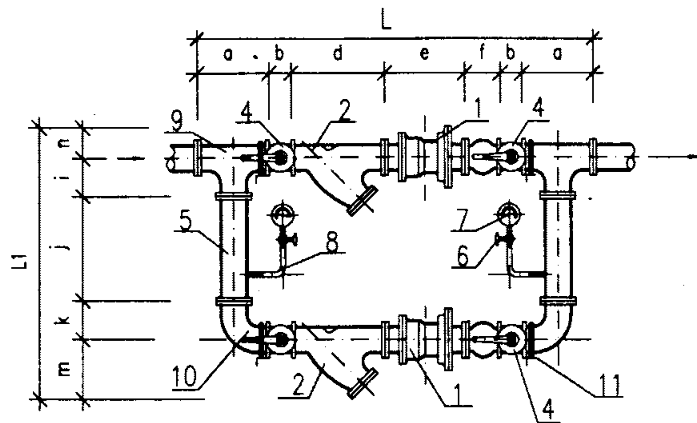
正视图
