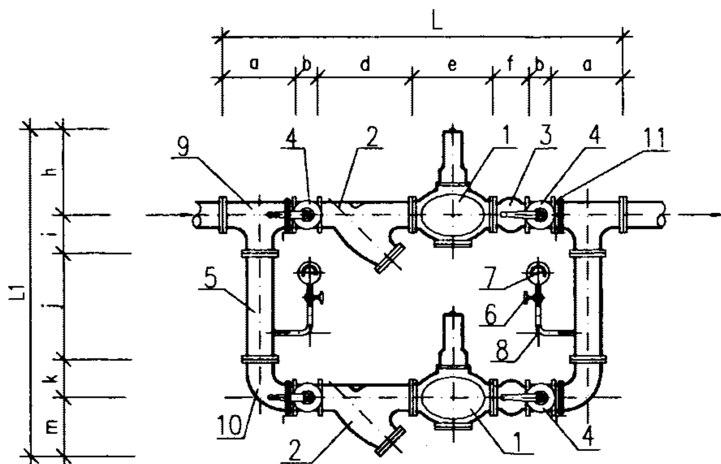
正视图
