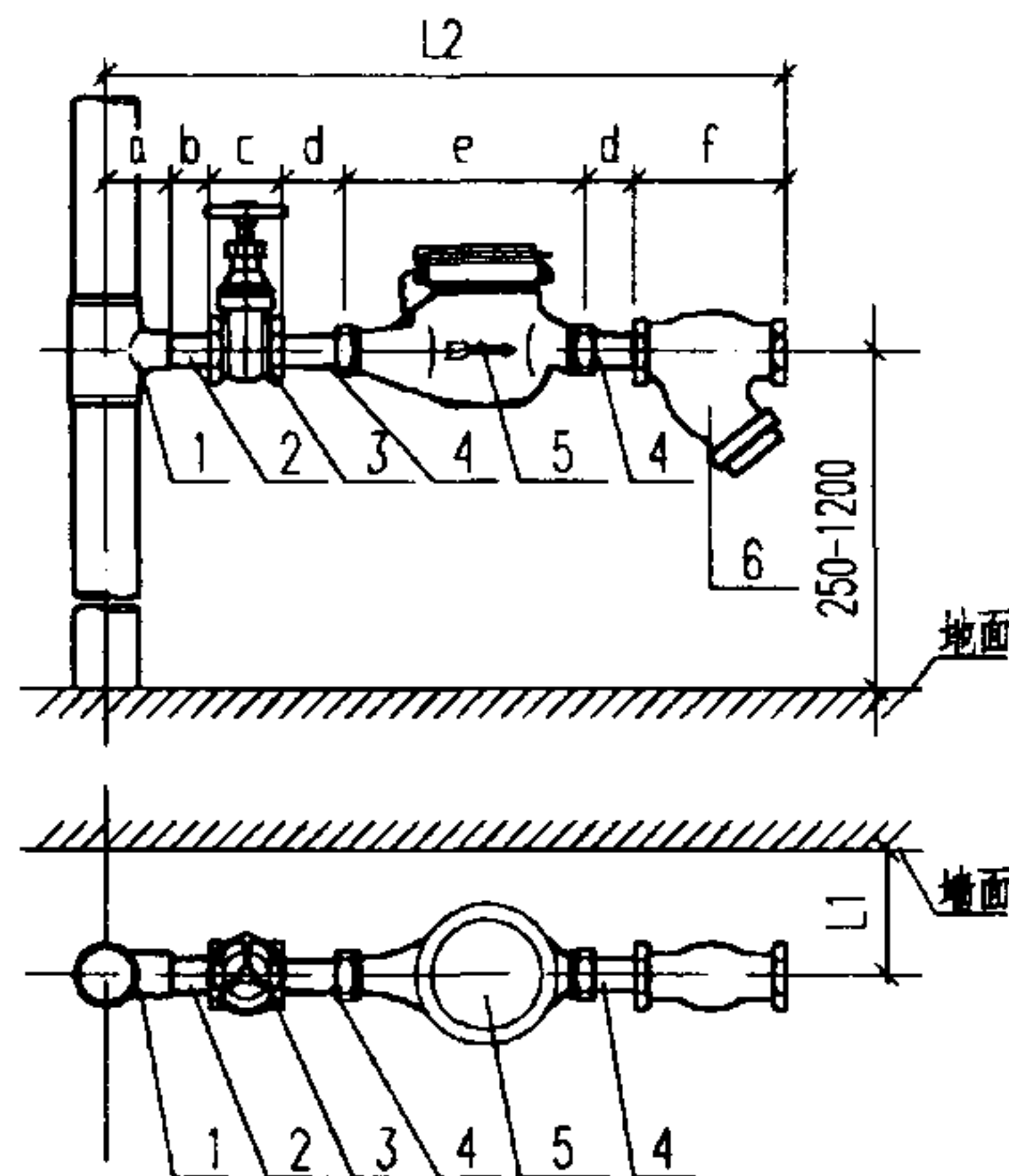
乙型安装图
