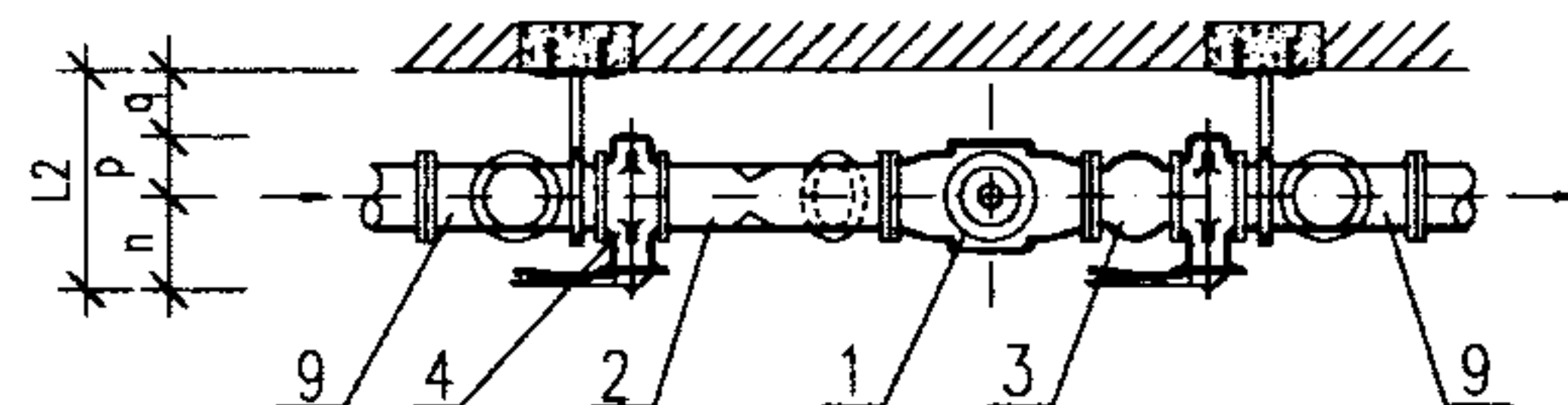
俯视图
