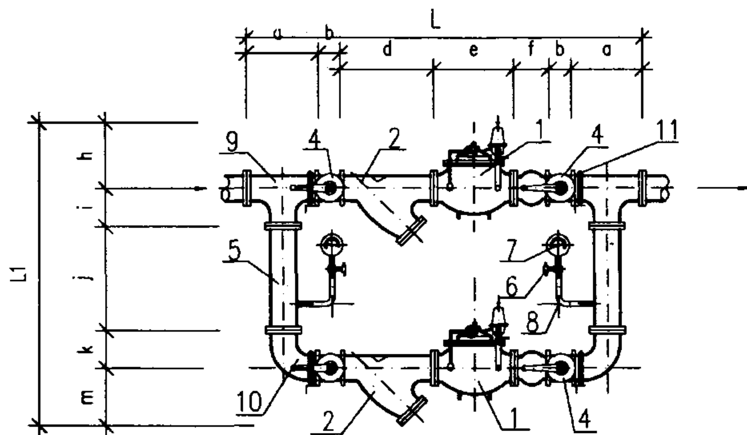
正视图
