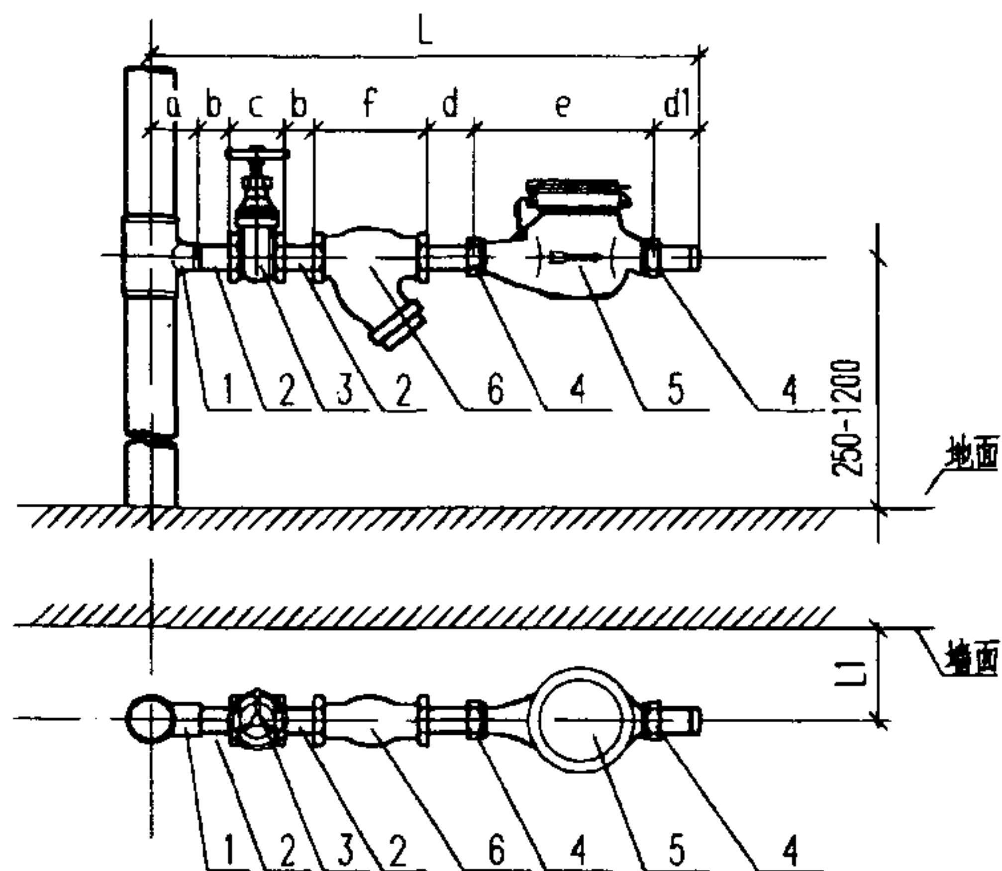
甲型安装图
