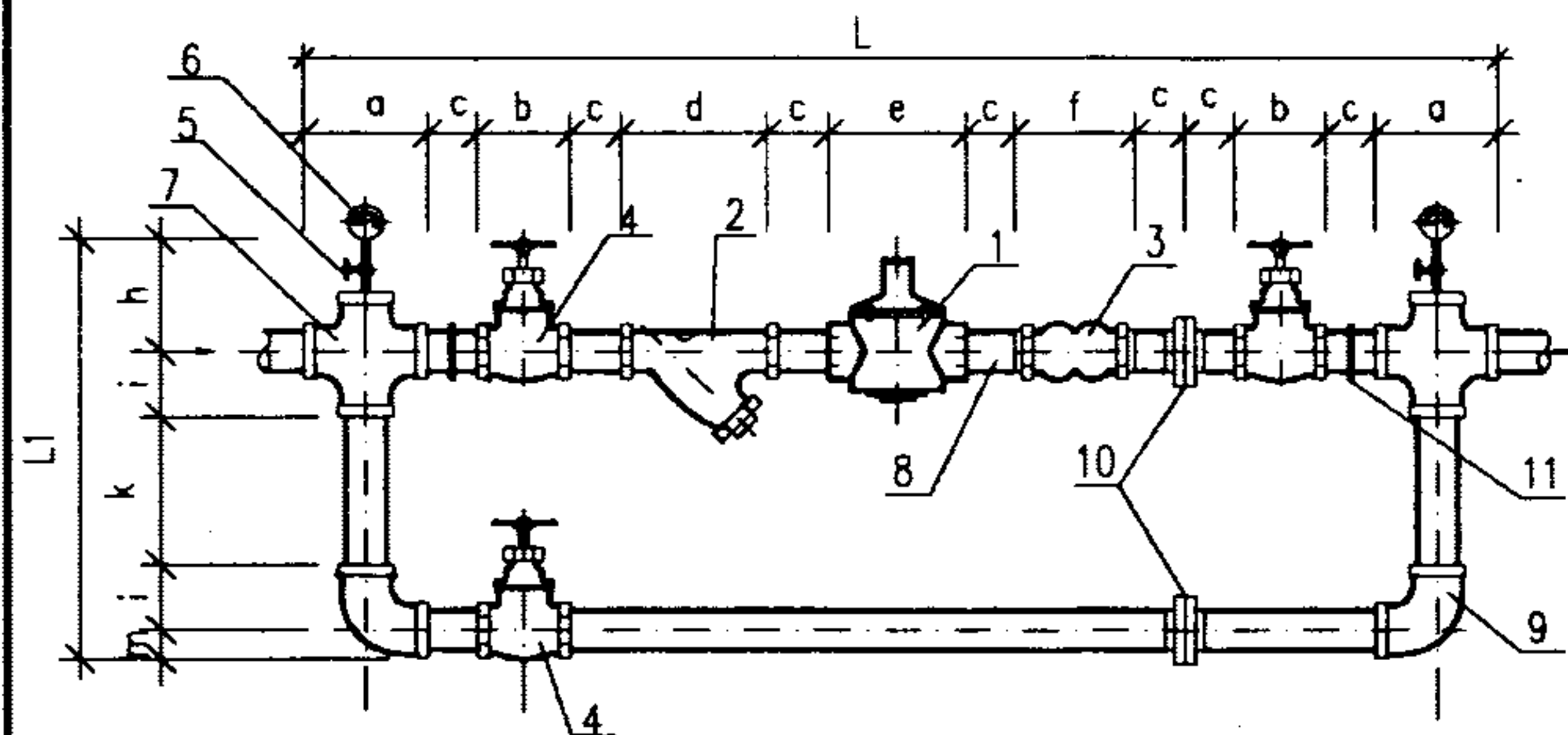
正视图
