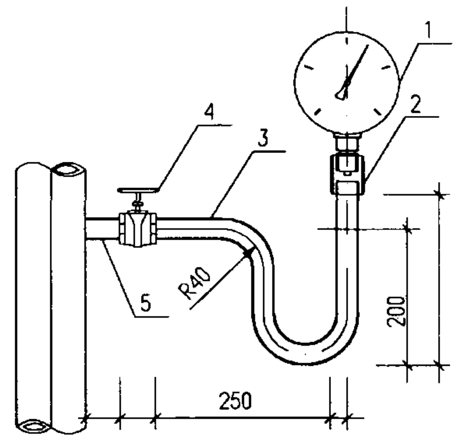
丁型
