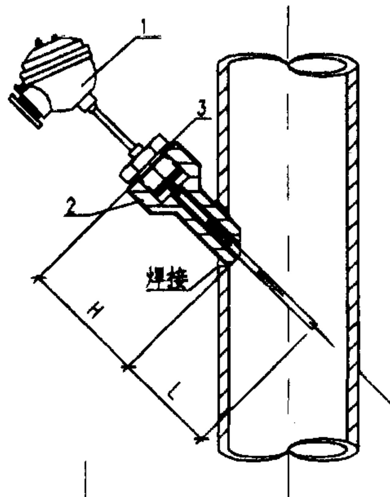
丙型
